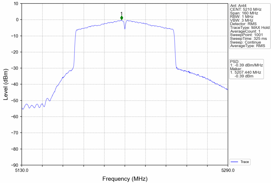
802.11ac(VHT80)_MCH_5210MHz_MIMO_NTNV
