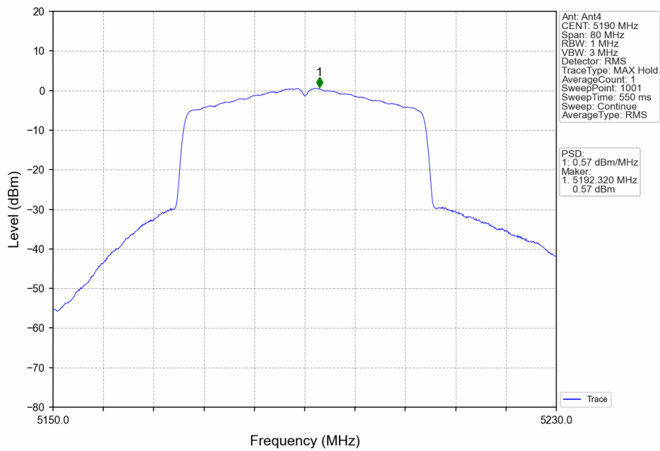
802.11ax(HEW40)_LCH_5190MHz_RU484_Left_Ant4_NTNV
