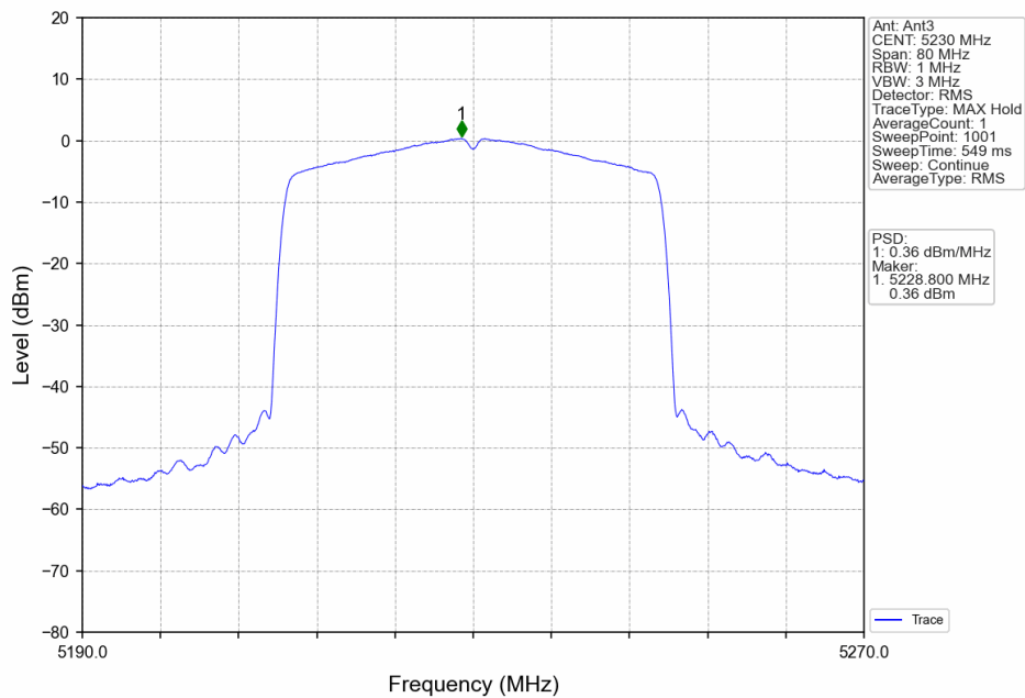
802.11ax(HEW40)_HCH_5230MHz_RU484_Left_Ant3_NTNV
