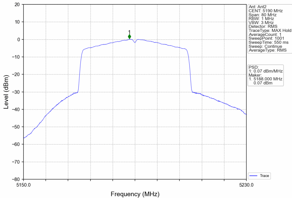
802.11ax(HEW40)_LCH_5190MHz_RU484_Left_Ant2_NTNV
