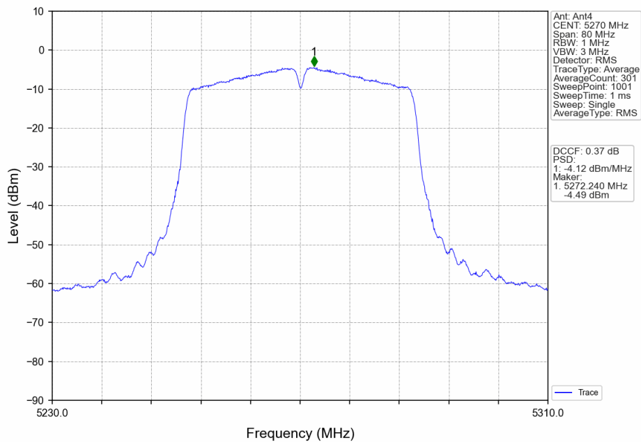
802.11n(HT40)_LCH_5270MHz_Ant4_NTNV
