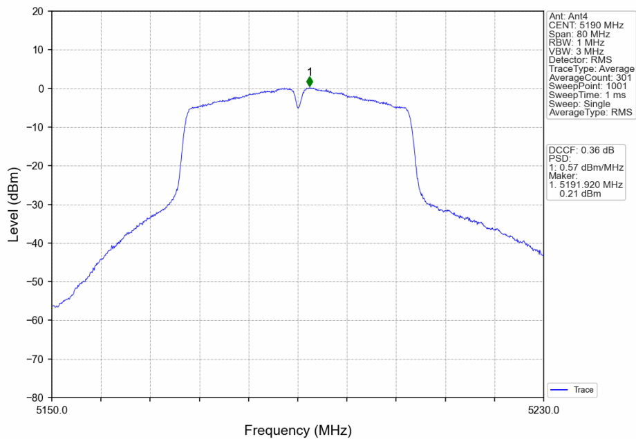
802.11n(HT40)_LCH_5190MHz_Ant4_NTNV
