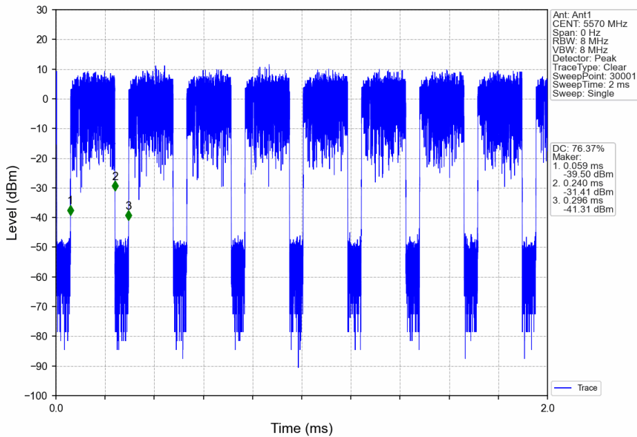
802.11ax(HEW160)_MCH_5570MHz_2xRU996_Left_Ant1_NTNV
