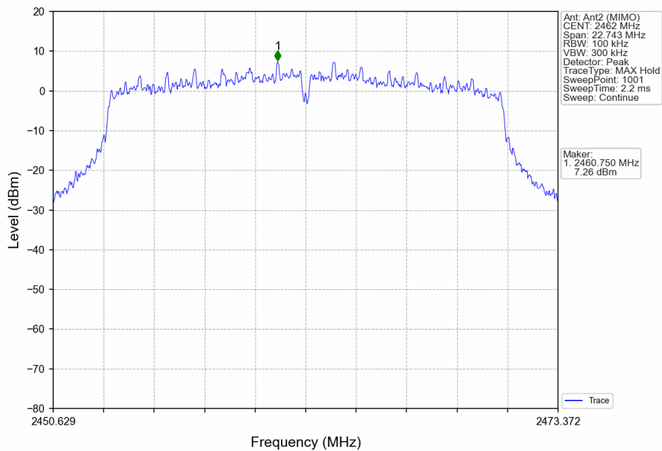
802.11ac(VHT20)_HCH_2462MHz_Ant2 (MIMO)_NTNV
