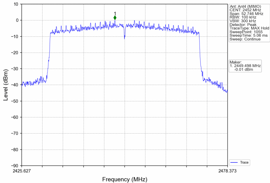
802.11ax(HEW40)_HCH_2452MHz_RU484_Left_Ant4 (MIMO)_NTNV
