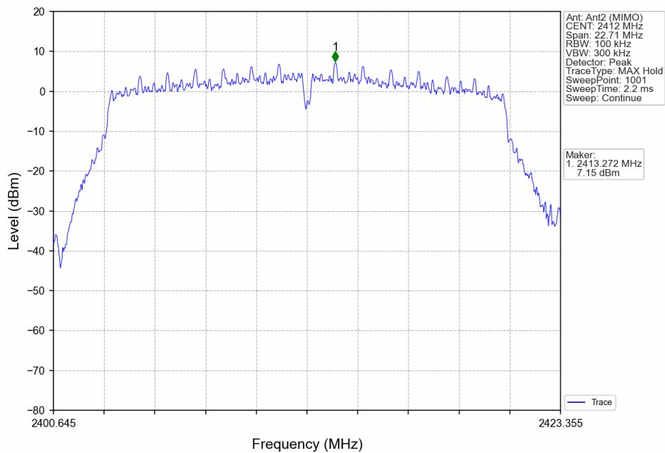
802.11ac(VHT20)_LCH_2412MHz_Ant2 (MIMO)_NTNV
