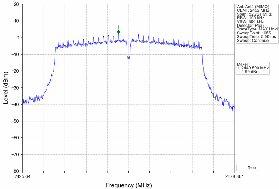
802.11n(HT40)_HCH_2452MHz_Ant4 (MIMO)_NTNV
