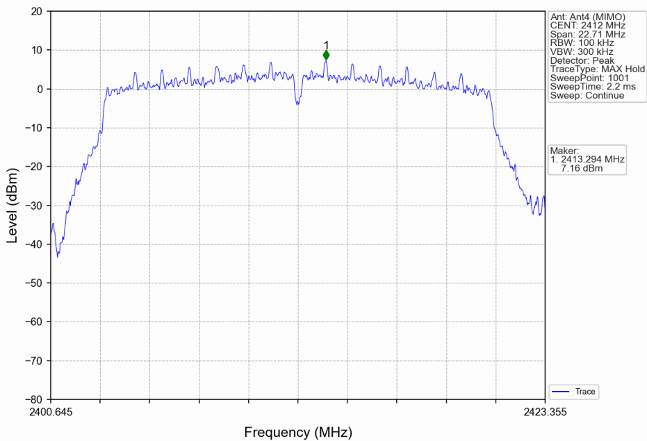
802.11ac(VHT20)_LCH_2412MHz_Ant4 (MIMO)_NTNV
