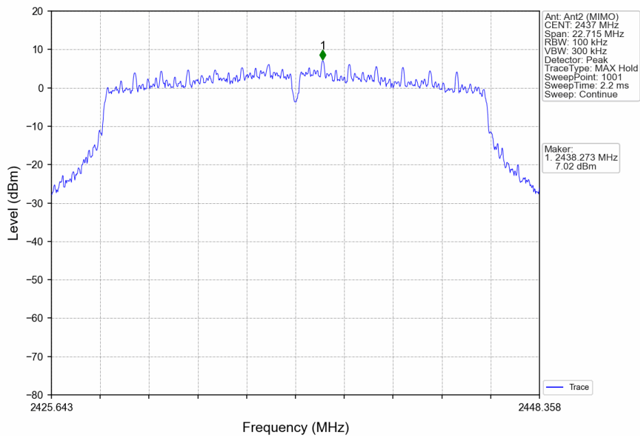
802.11ac(VHT20)_MCH_2437MHz_Ant2 (MIMO)_NTNV
