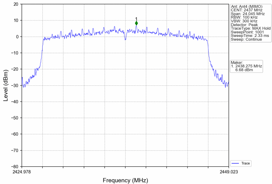
802.11ax(HEW20)_MCH_2437MHz_RU242_Left_Ant4 (MIMO)_NTNV
