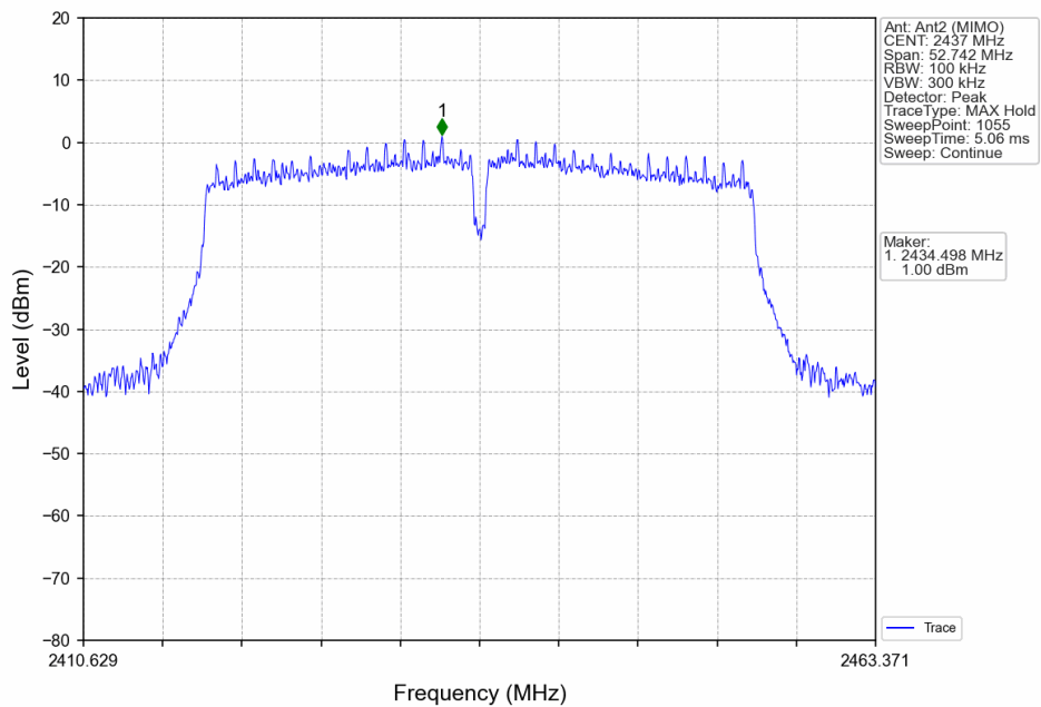
802.11ac(VHT40)_MCH_2437MHz_Ant2 (MIMO)_NTNV
