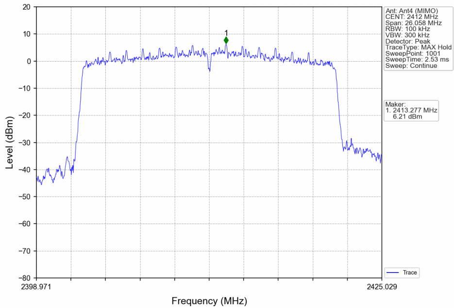
802.11ax(HEW20)_LCH_2412MHz_RU242_Left_Ant4 (MIMO)_NTNV
