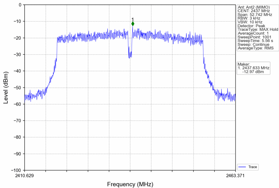
802.11ac(VHT40)_MCH_2437MHz_Ant2 (MIMO)_NTNV
