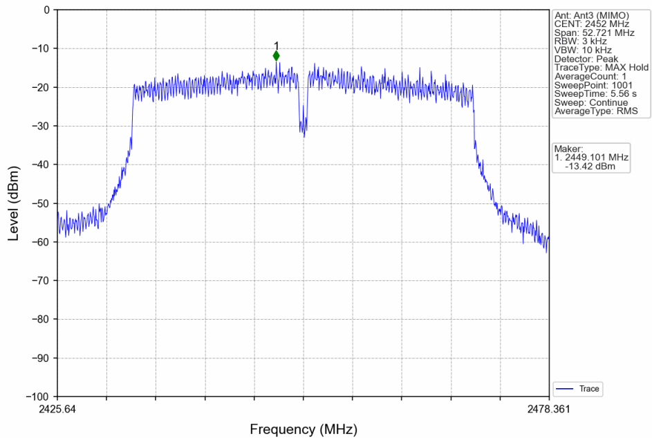
802.11n(HT40)_HCH_2452MHz_Ant3 (MIMO)_NTNV
