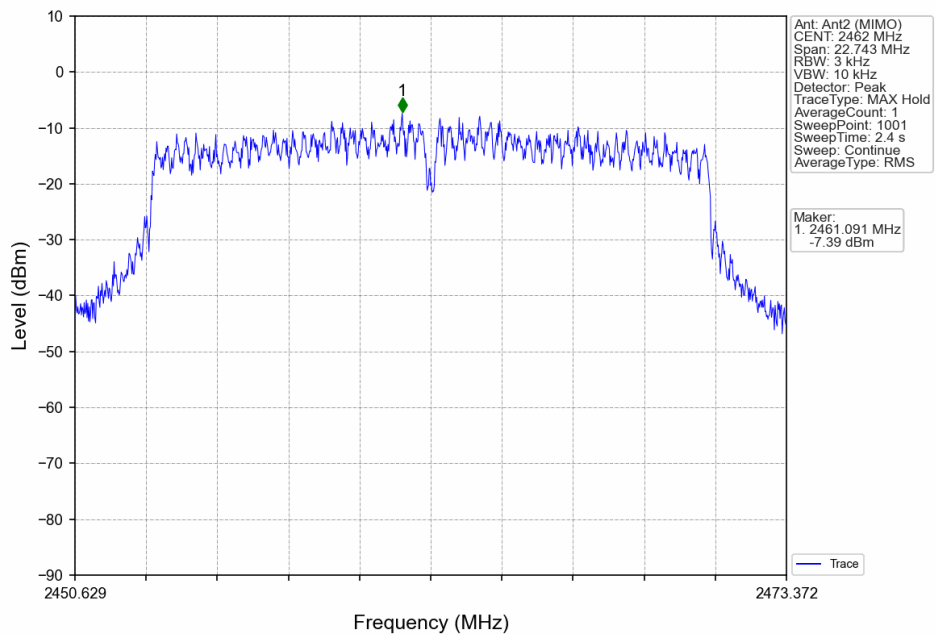
802.11ac(VHT20)_HCH_2462MHz_Ant2 (MIMO)_NTNV
