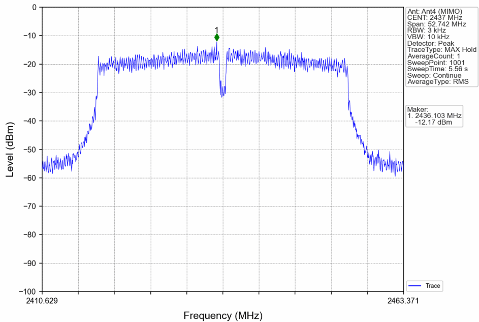
802.11ac(VHT40)_MCH_2437MHz_Ant4 (MIMO)_NTNV
