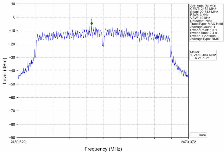
802.11ac(VHT20)_HCH_2462MHz_Ant4 (MIMO)_NTNV
