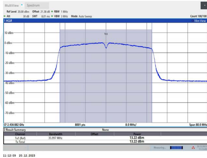
11N40MIMO_Ant2_2437
