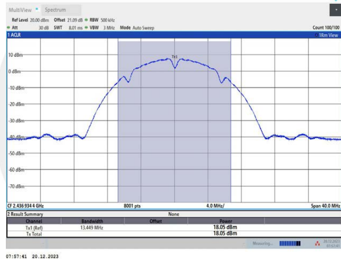
11B_Ant2_2437
