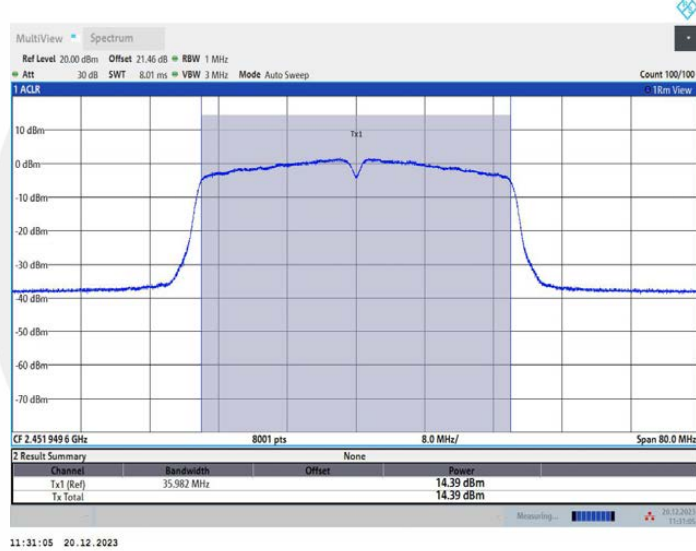
11N40MIMO_Ant4_2452
