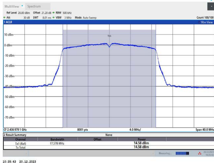
11N20MIMO_Ant3_2437
