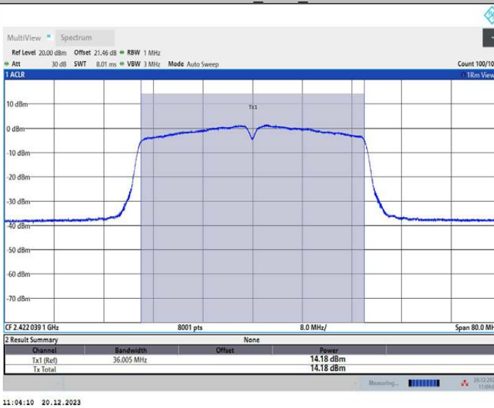
11N40MIMO_Ant4_2422
