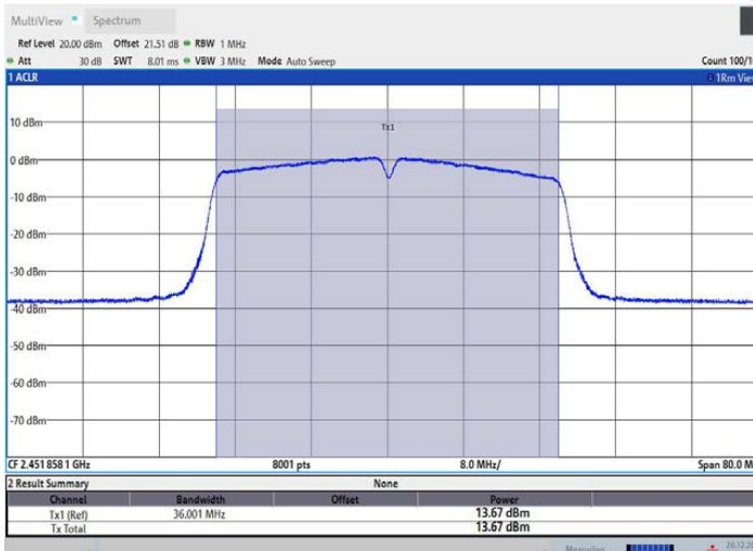
11N40MIMO_Ant2_2452
