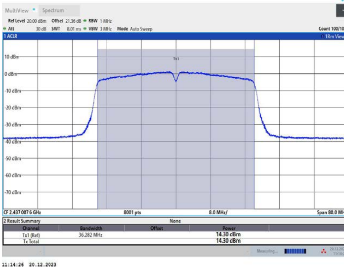
11N40MIMO_Ant3_2437
