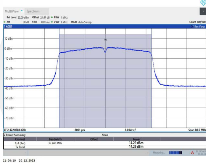
11N40MIMO_Ant3_2422
