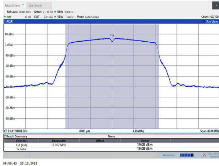
11G_Ant2_2412
