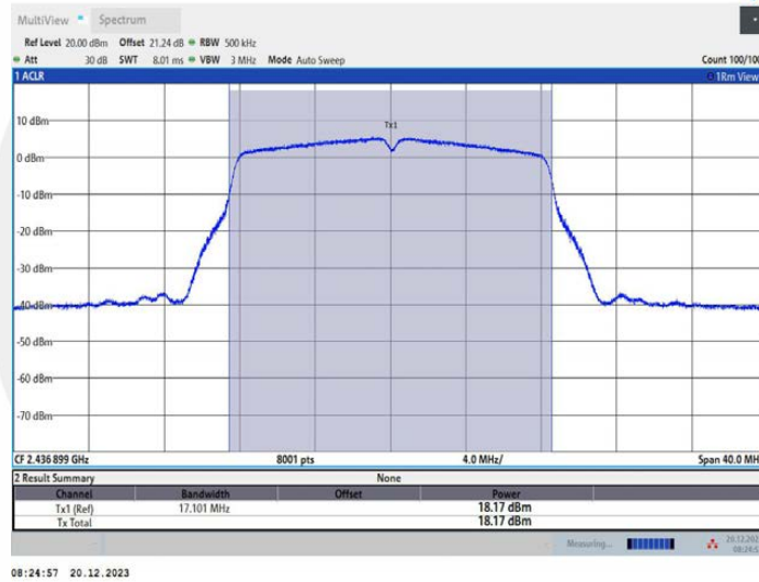
11G_Ant2_2437
