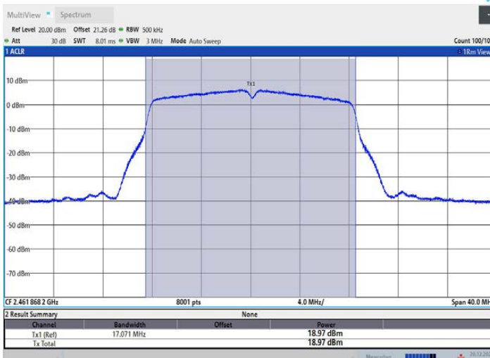
11G_Ant2_2462
