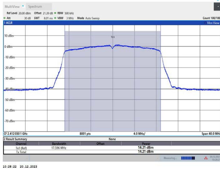
11N20MIMO_Ant4_2412
