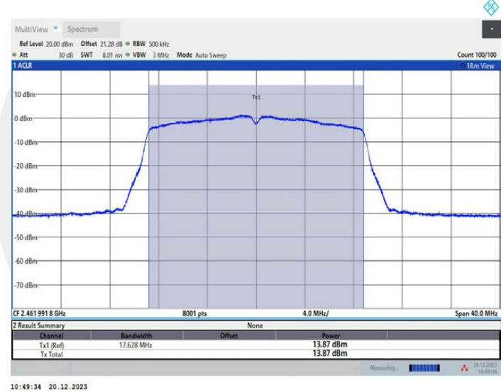
11N20MIMO Ant4 2462
