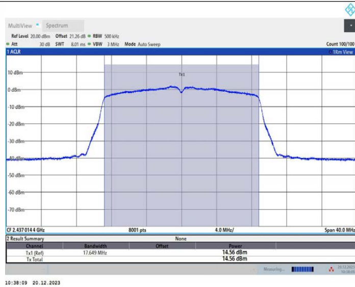
11N20MIMO_Ant4_2437
