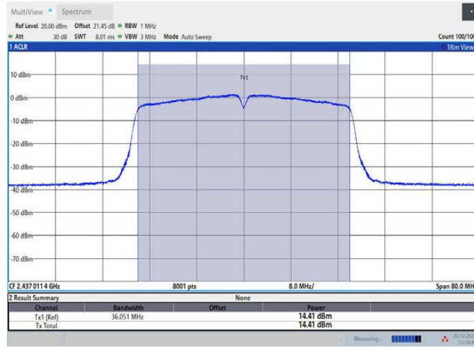
11N40MIMO_Ant4_2437
