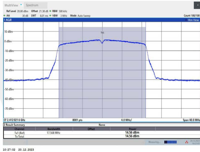
11N20MIMO_Ant3_2412
