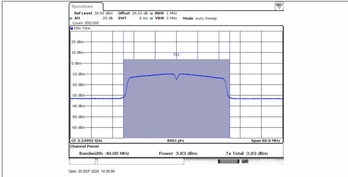
11N40MIMO_Ant2_5550
