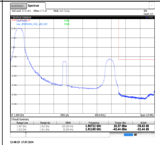
Band2-3MHz-QPSK-19185-1RB#14-PASS
