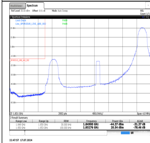
Band2-3MHz-QPSK-18615-15RB#0-PASS
