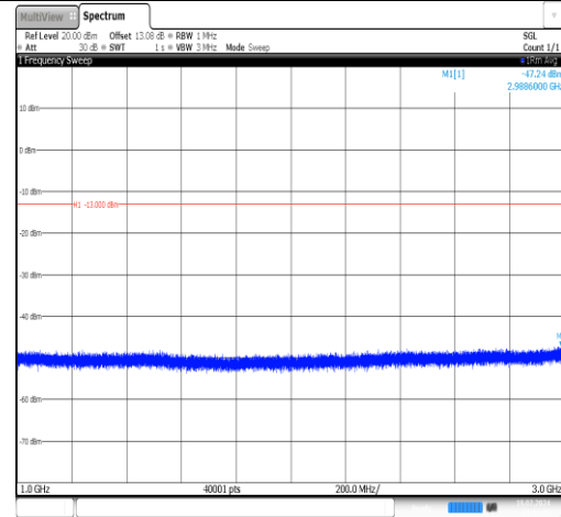
Band12-1.4MHz-QPSK-23017-1RB#5- 1000~3000-PASS
