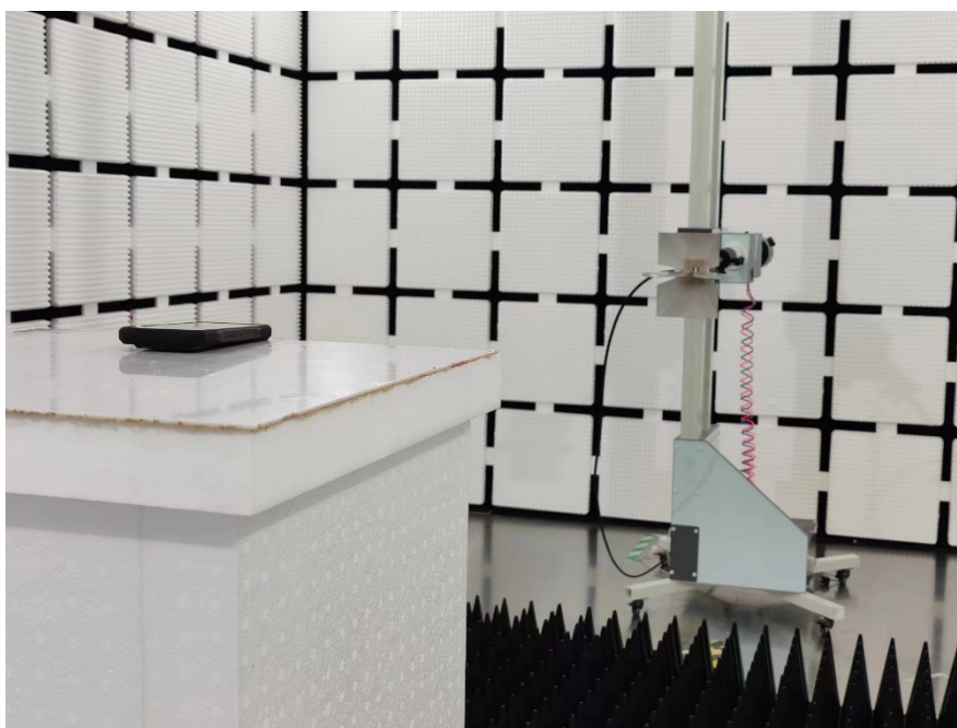
Above 1000MHz
