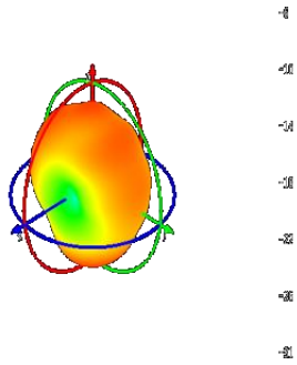
Ant0: 1575.42Mhz
