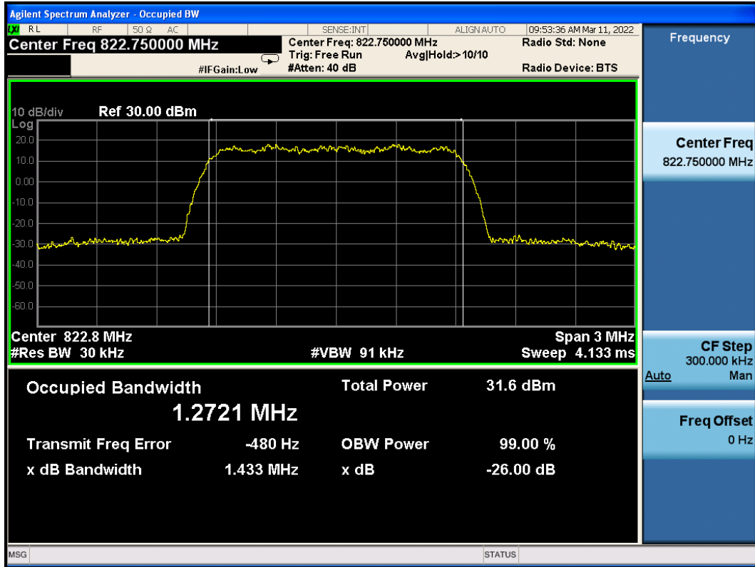
CDMA2000 BC10 1xEV-Do Rel.A Channel=450
