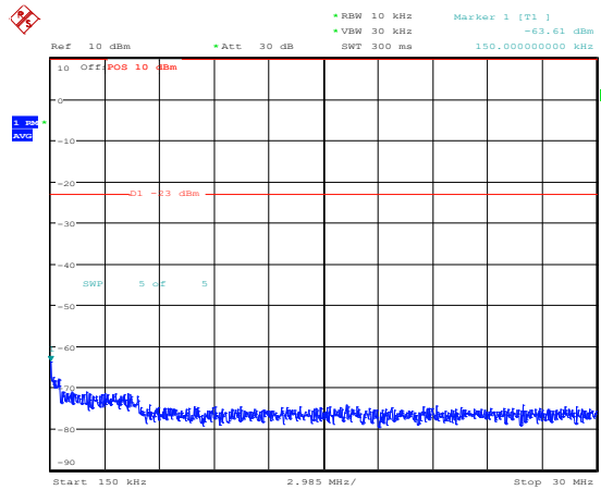
Band25-3MHz-QPSK-26365-1RB#0-Range2:0.15~30MHz
