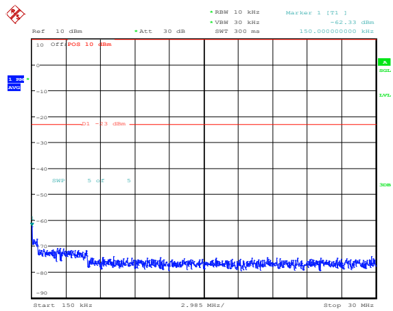
Band25-15MHz-QPSK-26115-1RB#0-Range2:0.15~30MHz
