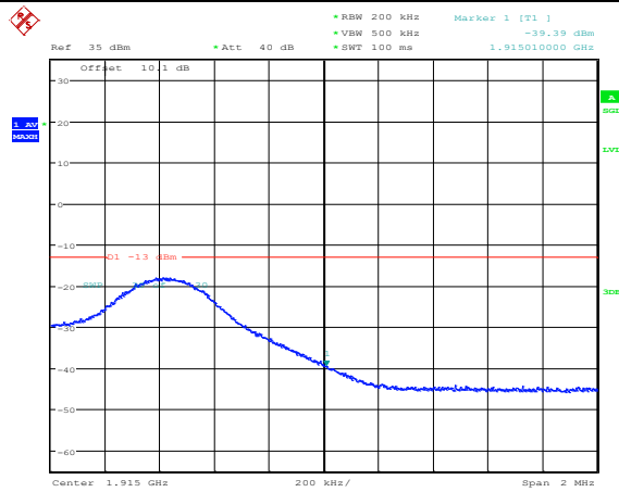
Band25-10MHz-QPSK-26640-1RB#0
