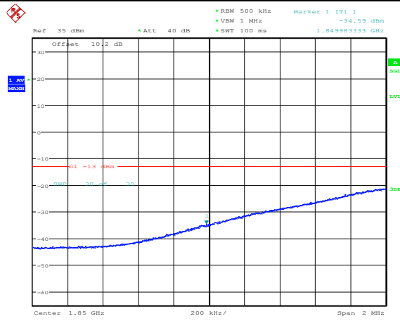
Band25-20MHz-QPSK-26140-1RB#99
