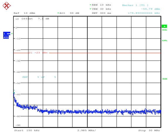
Band4-20MHz-QPSK-20175-1RB#0-Range2:0.15~30MHz
