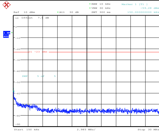
Band4-1.4MHz-QPSK-20175-1RB#0-Range2:0.15~30MHz
