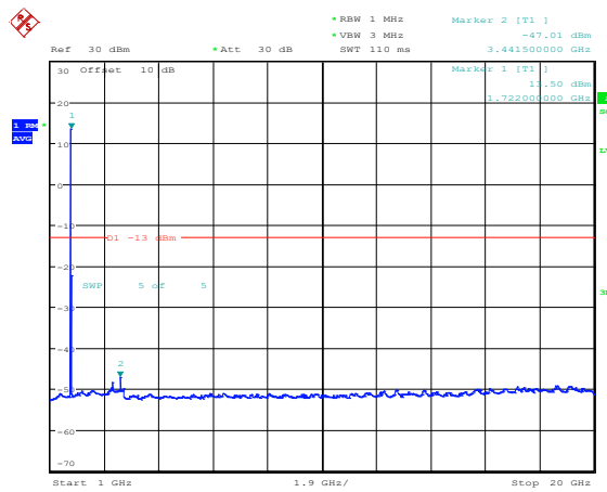
Band4-20MHz-QPSK-20175-1RB#0-Range4:1000~20000MHz
