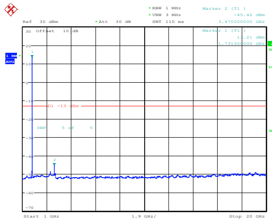
Band4-20MHz-QPSK-20300-1RB#0-Range4:1000~20000MHz
