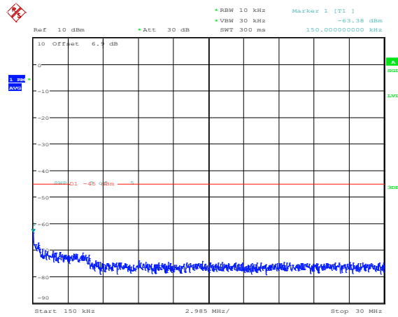
Band41-5MHz-QPSK-40265-1RB#0-Range2:0.15~30MHz
