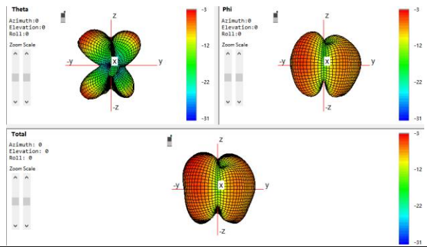
Aux: 1820Mhz
