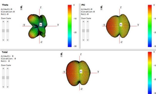
Aux: 2380Mhz
