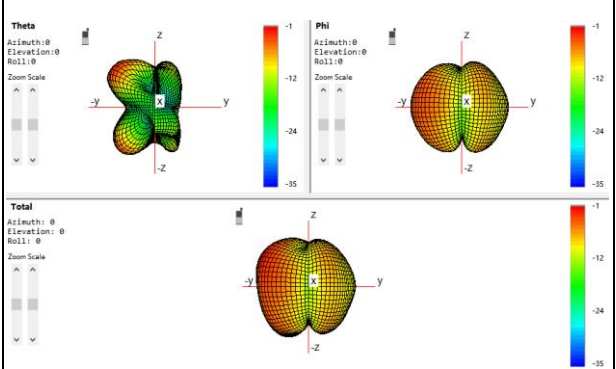
Aux: 2160Mhz
