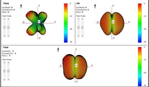
Aux: 1920Mhz
