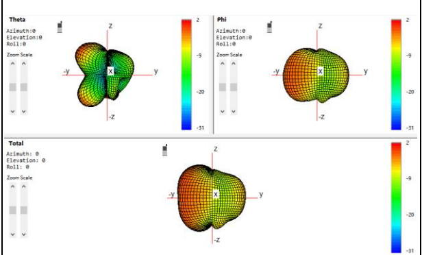
Aux: 2600Mhz
