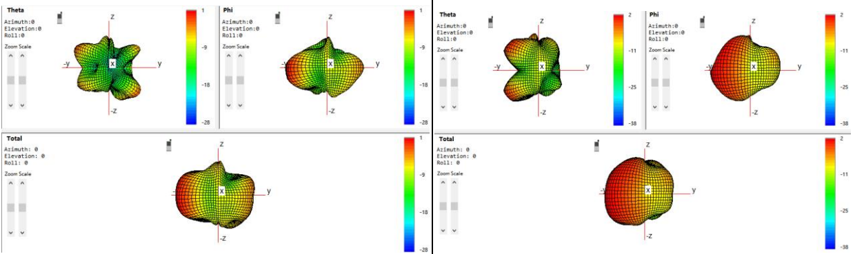
G/W/B: 5180Mhz
