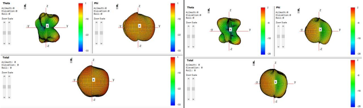
G/W/B: 1575Mhz
