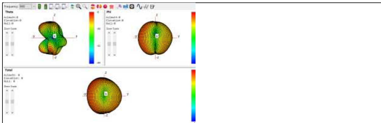
Aux: 960Mhz
