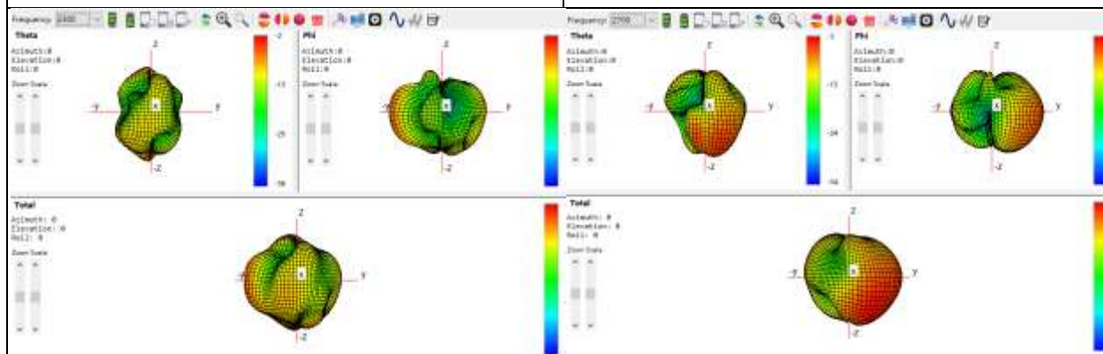
Aux: 2300Mhz
