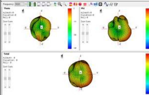
G/W/B: 5820Mhz
