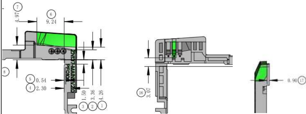
Ant1- GSM/WDMA/LTE div: Monopole
