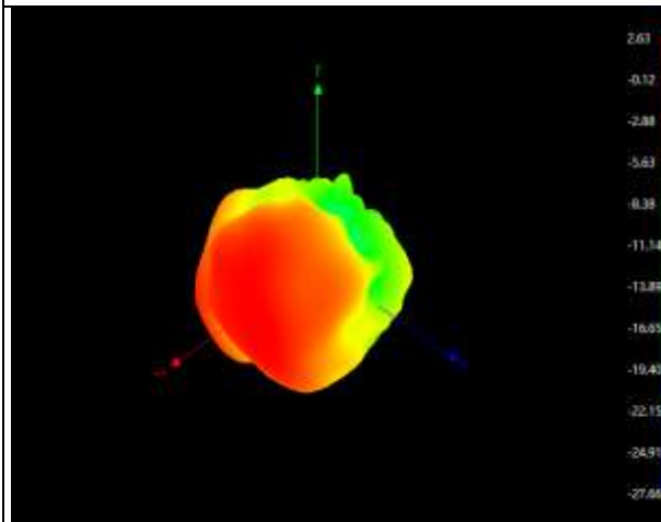
Ant0: 1900Mhz
