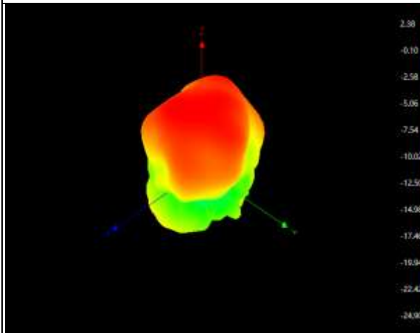
Ant0: 900Mhz
