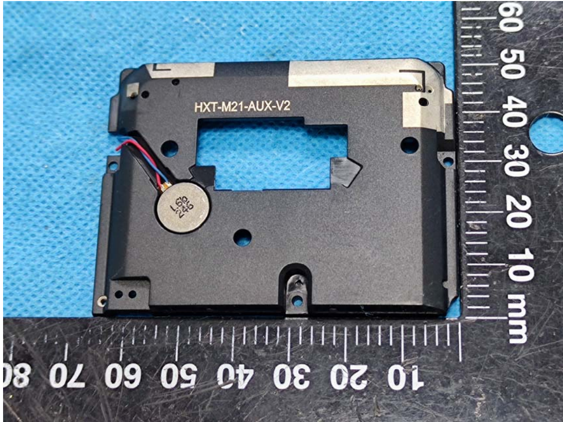
Bluetooth/WiFi Antenna WWAN Aux Antenna
