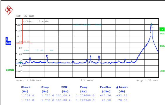
Band66_20MHz_QPSK_132072_1RB#0
