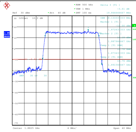
Band25-20MHz-16QAM-26365-100RB#0-PASS
