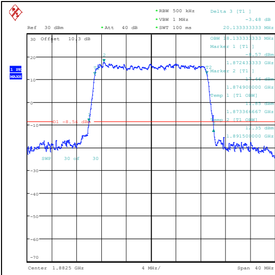
Band25-20MHz-QPSK-26365-100RB#0-PASS
