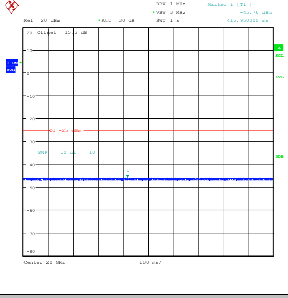
Band41(2535-2655)-10MHz-16QAM-41190-1RB#0 -20000~27000-PASS
