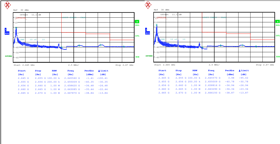
Band41_10MHz_QPSK_41190_1RB#0
