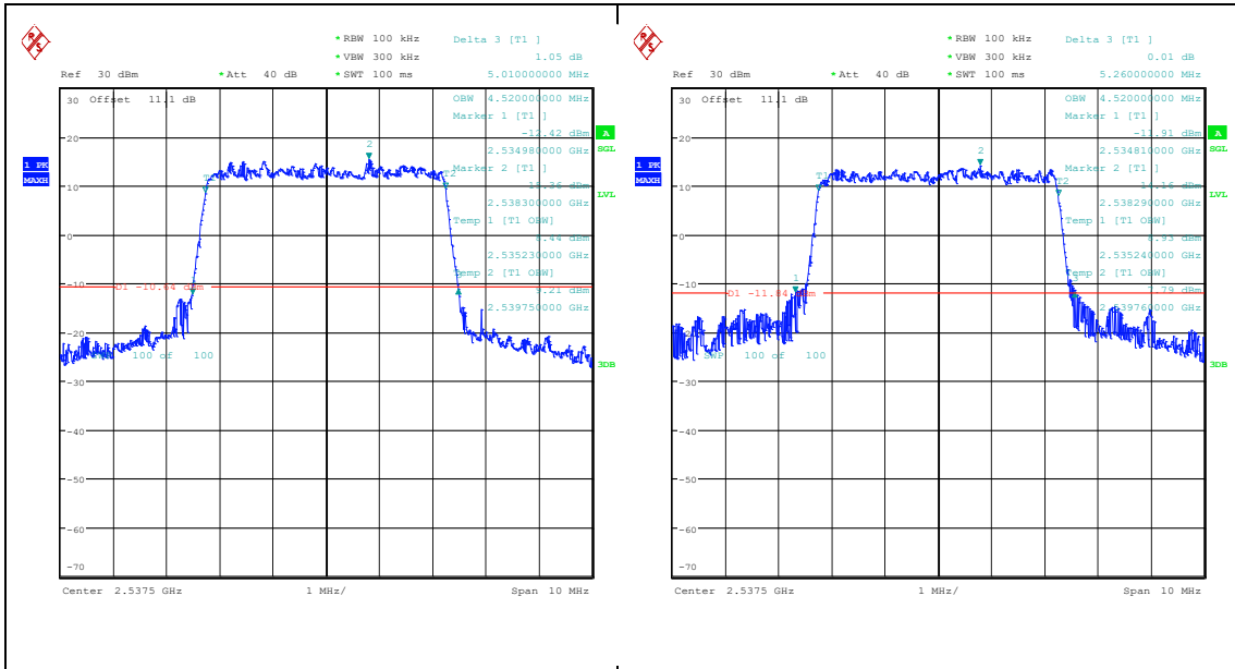
Band41(2535-2655)-5MHz-QPSK-40065-25RB#0 -PASS Band41(2535-2655)-5MHz-16QAM-40065-25RB#0 -PASS
