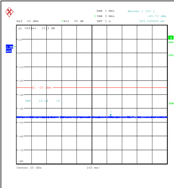
Band41(2535-2655)-10MHz-QPSK-40590-1RB#0 -20000~27000-PASS
