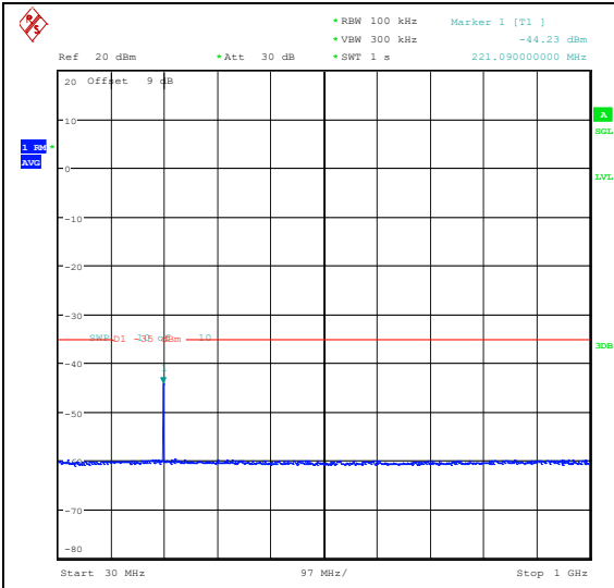
Band41(2535-2655)-10MHz-QPSK-40090-1RB#0 -30~1000-PASS
