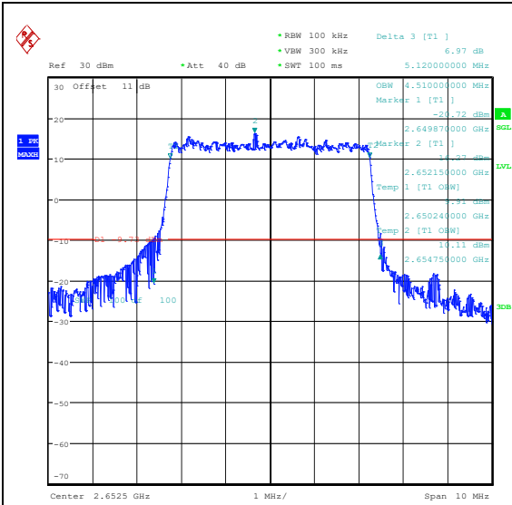
Band41(2535-2655)-5MHz-QPSK-41215-25RB#0 -PASS
