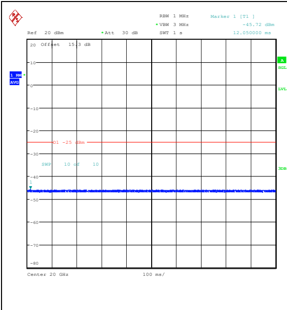
Band41(2535-2655)-5MHz-QPSK-40065-1RB#0-2000~27000-PASS
