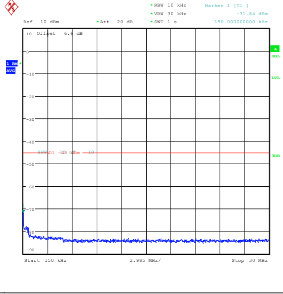
Band41(2535-2655)-10MHz-QPSK-41190-1RB#0- 0.15-30-PASS
