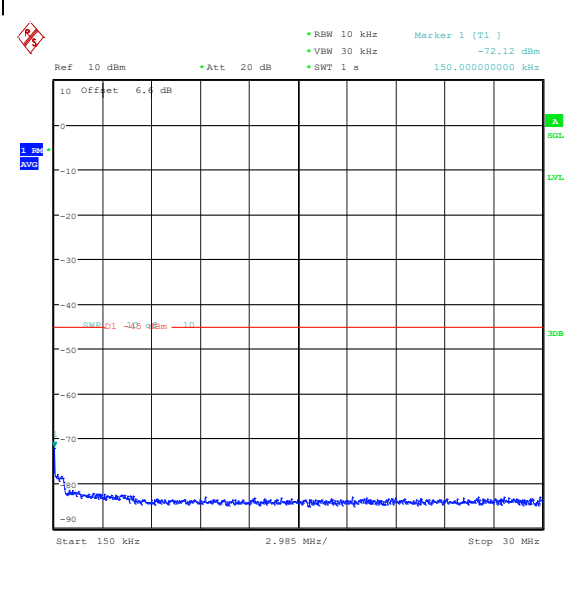
Band41(2535-2655)-5MHz-QPSK-40590-1RB#0-0. 15~30-PASS
