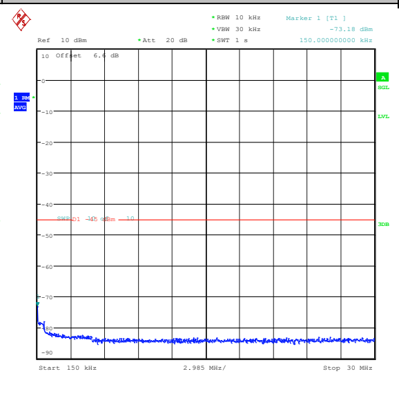
Band41(2535-2655)-10MHz-QPSK-40090-1RB#0- 0.15~30-PASS
