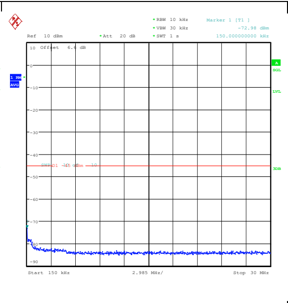
Band41(2535-2655)-10MHz-QPSK-40590-1RB#0- 0.15~30-PASS
