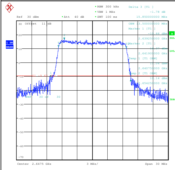
Band41(2535-2655)-15MHz-QPSK-41165-75RB#
