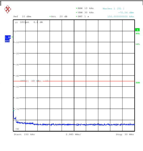
Band41(2535-2655)-20MHz-QPSK-40590-1RB#0- 0.15~30-PASS
