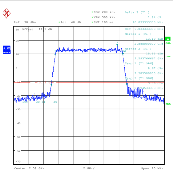
Band41(2535-2655)-10MHz-16QAM-40590-50RB# 0-PASS
