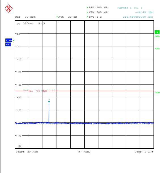
Band41(2535-2655)-20MHz-QPSK-40590-1RB#0 -30~1000-PASS
