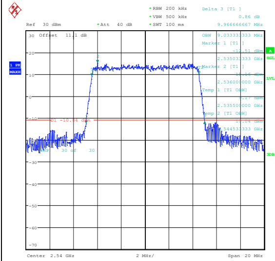
Band41(2535-2655)-10MHz-QPSK-40090-50RB#0 0-PASS
