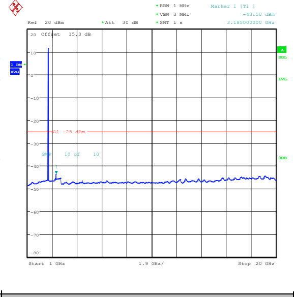
Band41(2535-2655)-10MHz-QPSK-40590-1RB#0- 1000~20000-PASS
