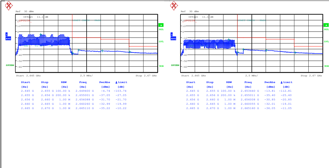
Band41_10MHz_QPSK_41190_50RB#0
