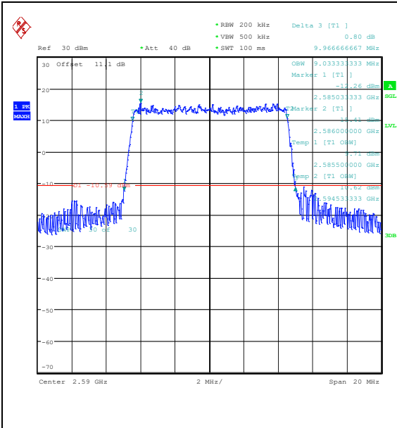
Band41(2535-2655)-10MHz-QPSK-40590-50RB# 0-PASS
