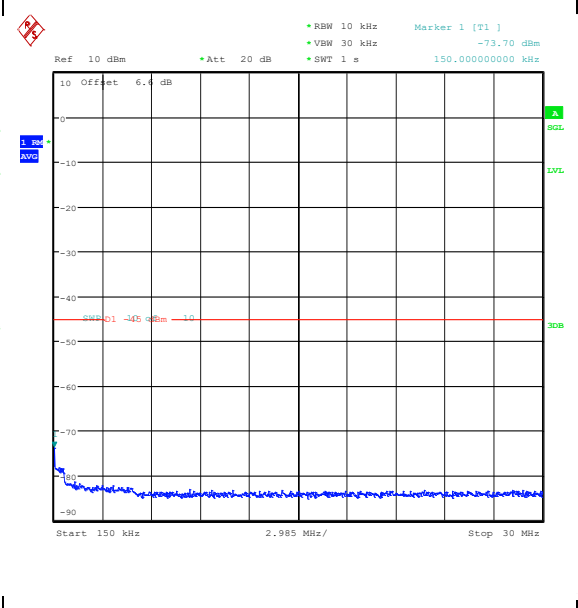
Band41(2535-2655)-20MHz-QPSK-41140-1RB#0- 0.15~30-PASS
