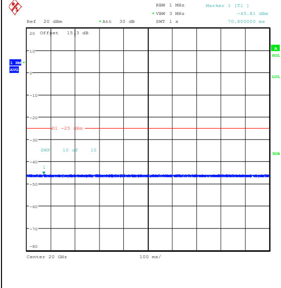
Band41(2535-2655)-10MHz-QPSK-41190-1RB#0-20000~27000-PASS
