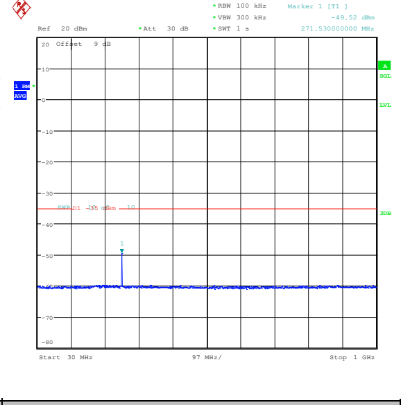
Band41(2535-2655)-10MHz-16QAM-40590-1RB#0 -30~1000-PASS
