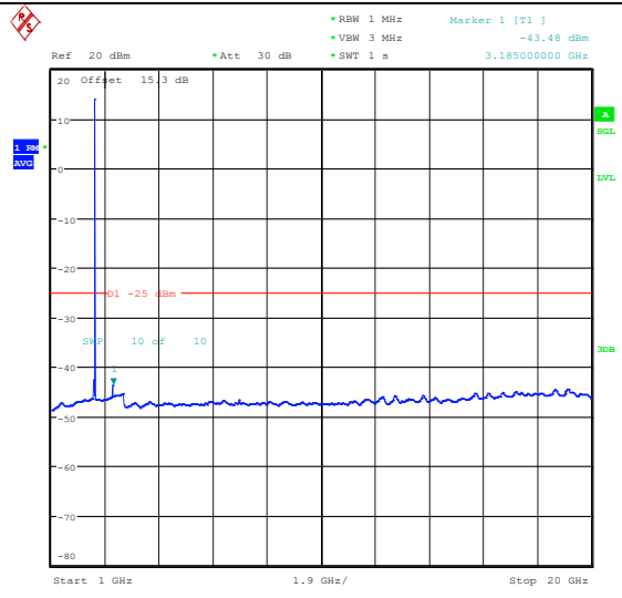
Band41(2535-2655)-10MHz-QPSK-40090-1RB#0- 1000~20000-PASS
