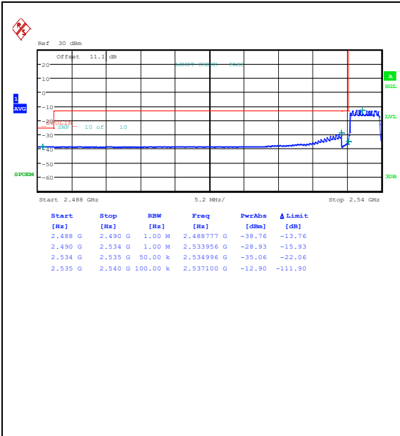
Band41_5MHz_QPSK_40065_25RB#0
