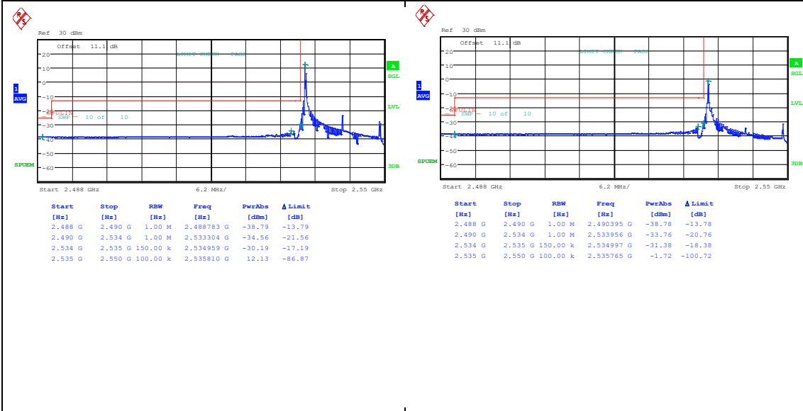
Band41_15MHz_QPSK_40115_1RB#0
