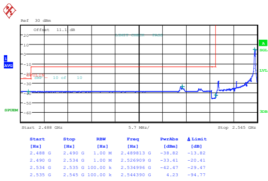
Band41_10MHz_QPSK_40090_1RB#0
