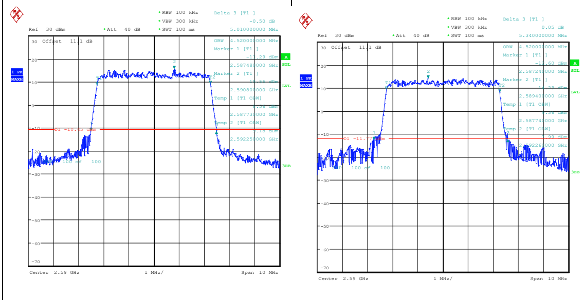
Band41(2535-2655)-5MHz-QPSK-40590-25RB#0 -PASS Band41(2535-2655)-5MHz-16QAM-40590-25RB#0 -PASS
