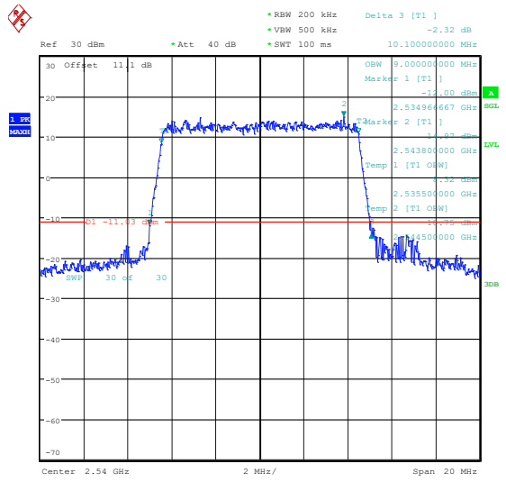
Band41(2535-2655)-10MHz-16QAM-40090-50RB#0 0-PASS
