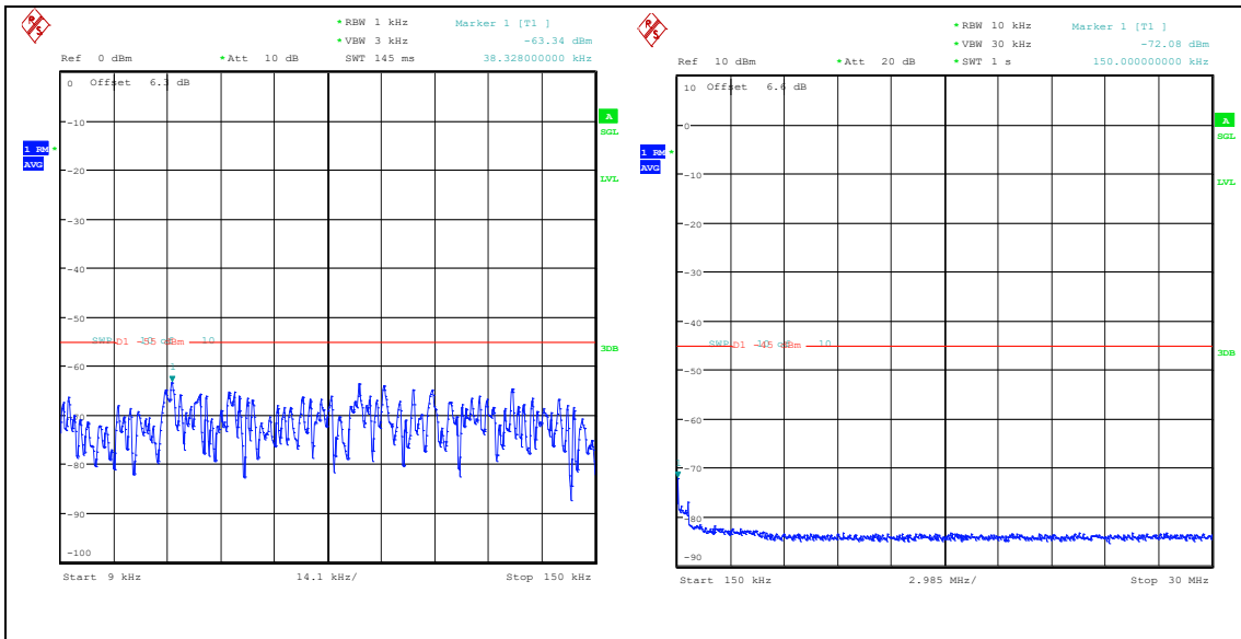
Band41(2535-2655)-5MHz-QPSK-40065-1RB#0-0.009~0.15-PASS
