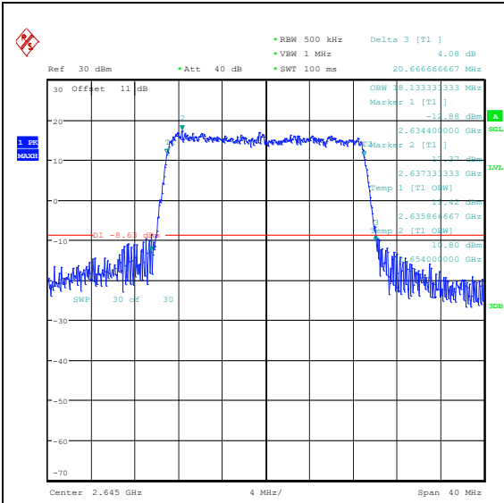
Band41(2535-2655)-20MHz-QPSK-41140-100RB #0-PASS
