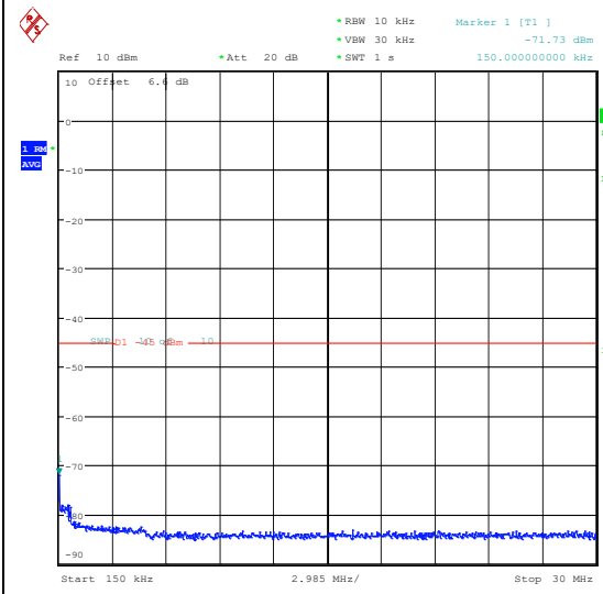
Band41(2535-2655)-20MHz-QPSK-40590-1RB#0 -20000~27000-PASS
