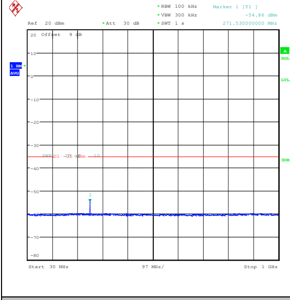
Band41(2535-2655)-10MHz-QPSK-40590-1RB#0 -30~1000-PASS
