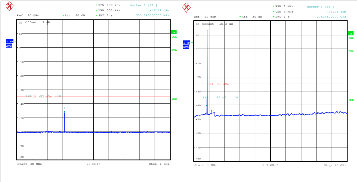
Band41(2535-2655)-10MHz-QPSK-41190-1RB#0-30~1000-PASS
