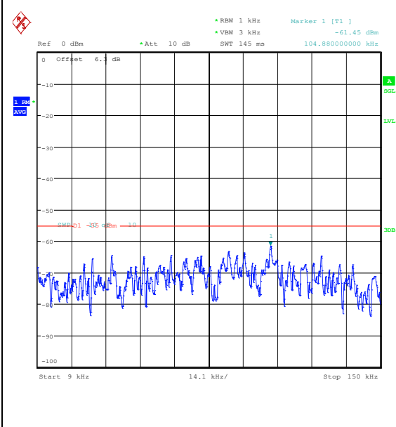
Band41(2535-2655)-20MHz-QPSK-41140-1RB#0- 0.009~0.15-PASS
