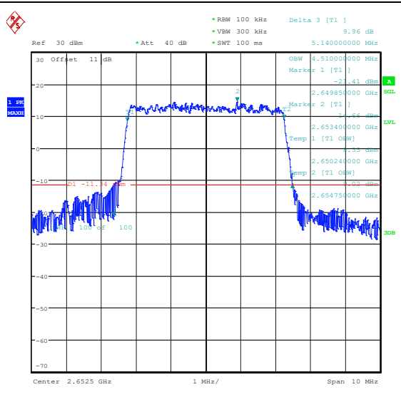
Band41(2535-2655)-5MHz-16QAM-41215-25RB#0 -PASS
