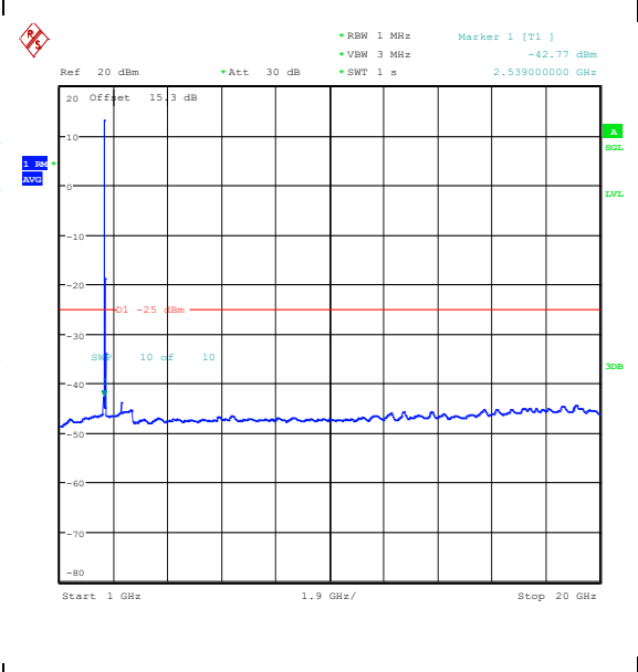
Band41(2535-2655)-20MHz-QPSK-40590-1RB#0- 1000~20000-PASS
