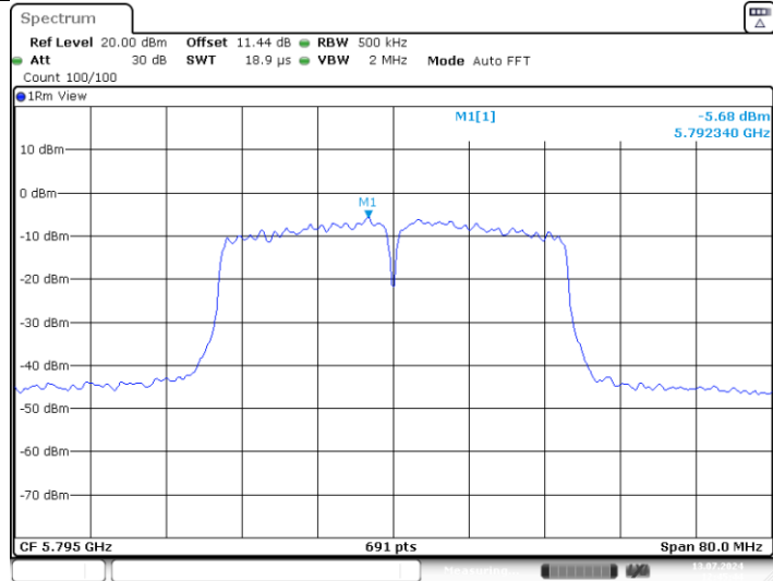
11N40MIMO_Ant1_5795
