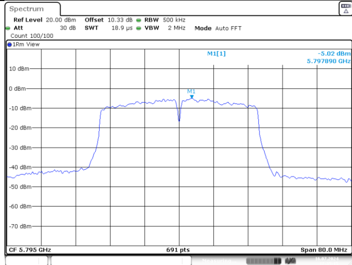
11N40MIMO_Ant2_5795
