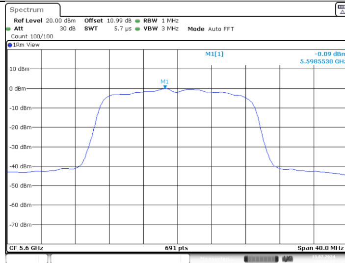
11N20MIMO_Ant1_5600
