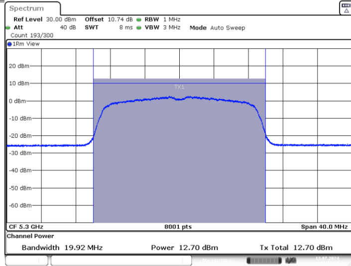
11AX20MIMO_Ant2_5300
