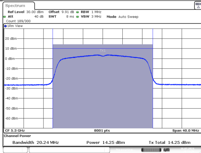
11AX20MIMO_Ant2_5300
