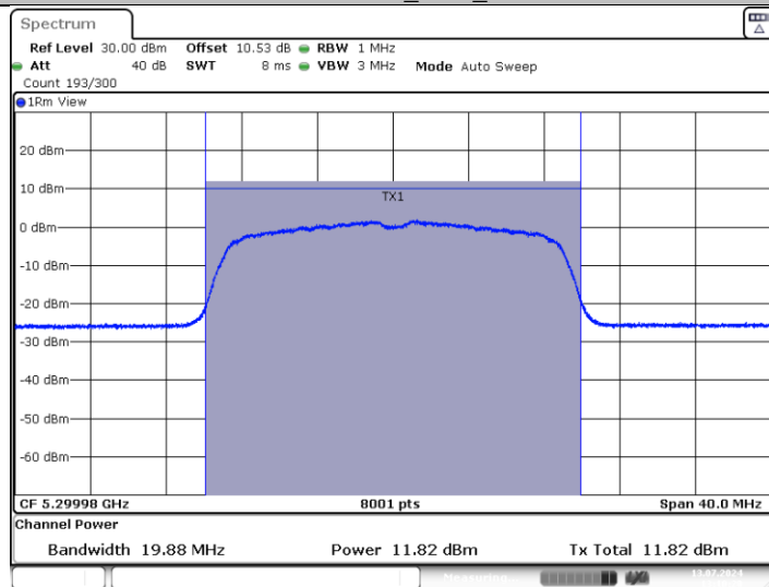
11AC20MIMO_Ant1_5300
