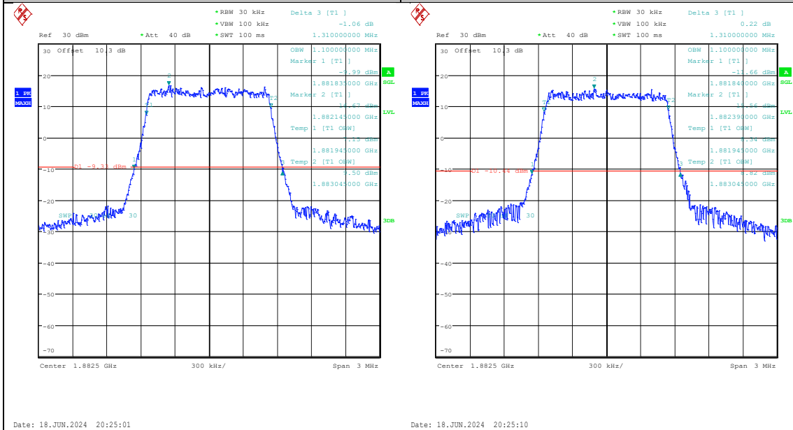
Band25-1.4MHz-QPSK-26365-6RB#0-PASS Band25-1.4MHz-16QAM-26365-6RB#0-PASS
