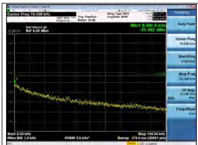
GSM1900-661-0-0.009~0.15MHz
