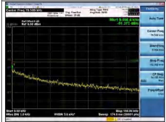
GPRS1900-810-0-0.009~0.15MHz
