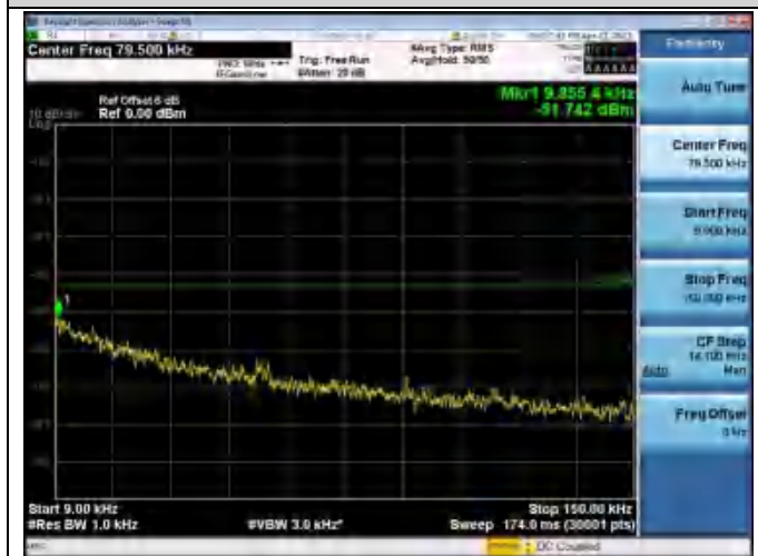
GPRS1900-512-0-0.009~0.15MHz
