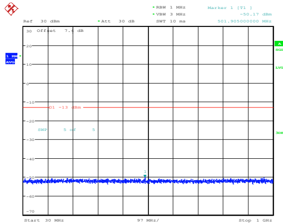
Band66-20MHz-QPSK-132072-1RB#0-Range3:30~1000MHz
