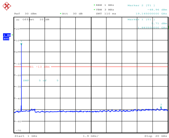
Band2-20MHz-QPSK-19100-1RB#0-Range4:1000~20000MHz
