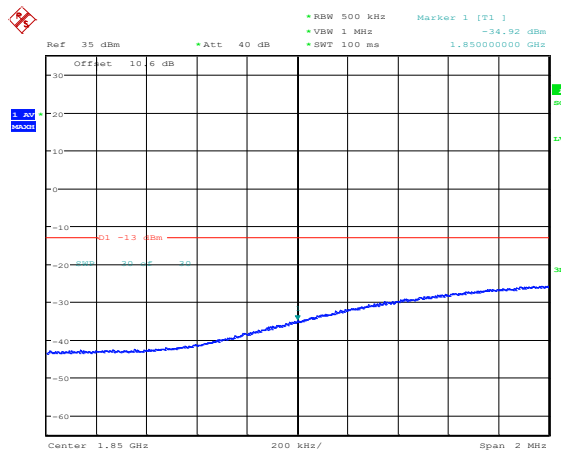
Band2-20MHz-QPSK-18700-1RB#99
