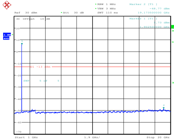
Band2-5MHz-16QAM-19175-1RB#0-Range4:1000~20000MHz
