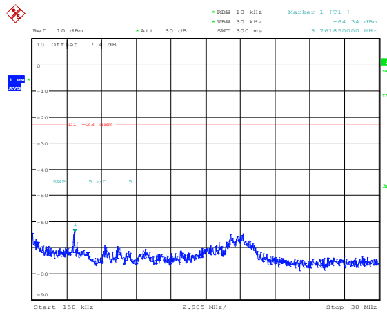
Band2-20MHz-16QAM-18700-1RB#0-Range2:0.15~30MHz
