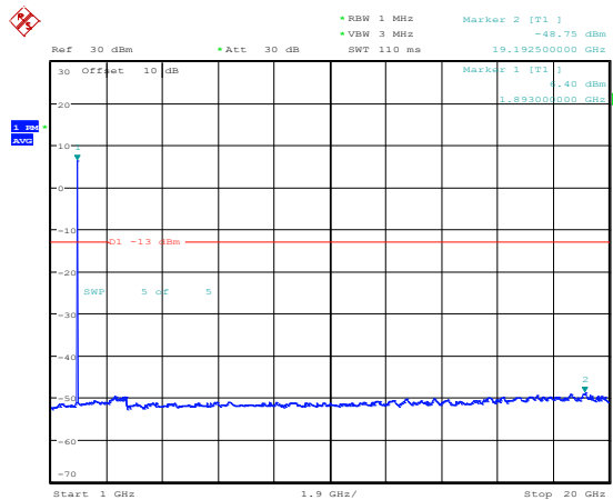
Band2-15MHz-QPSK-19125-1RB#0-Range4:1000~20000MHz
