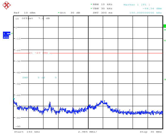
Band2-20MHz-16QAM-18900-1RB#0-Range2:0.15~30MHz
