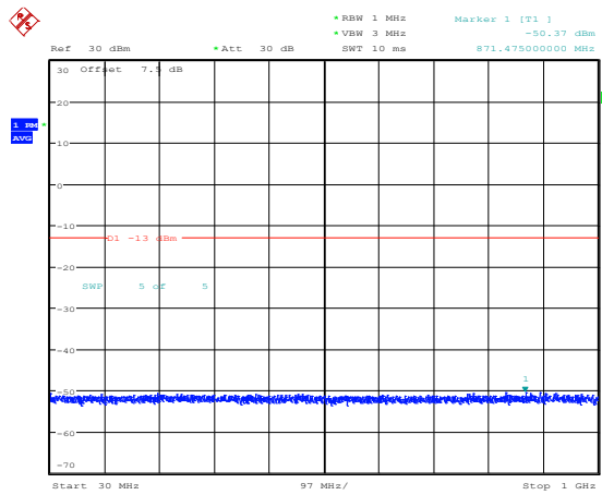
Band2-20MHz-QPSK-19100-1RB#0-Range3:30~1000MHz
