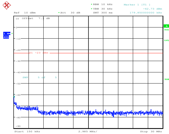
Band25-20MHz-QPSK-26140-1RB#0-Range2:0.15~30MHz
