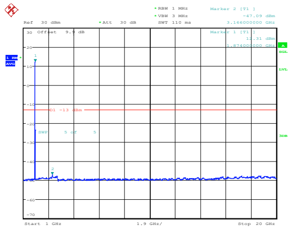
Band25-5MHz-QPSK-26365-1RB#0-Range4:1000~20000MHz
