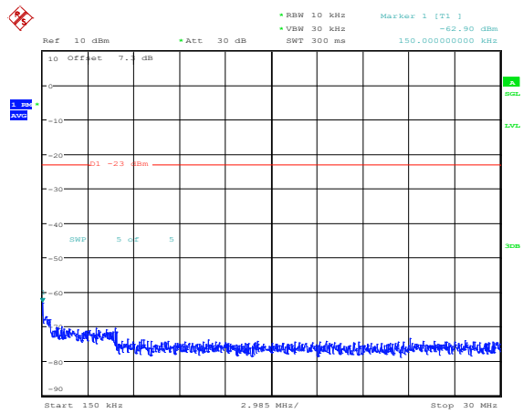
Band25-10MHz-QPSK-26090-1RB#0-Range2:0.15~30MHz
