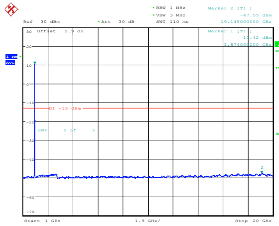
Band25-20MHz-16QAM-26365-1RB#0-Range4:1000~20000MHz
