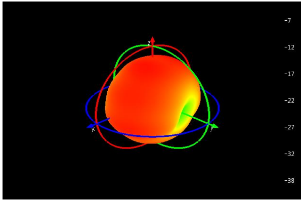
Ant0: 700Mhz
