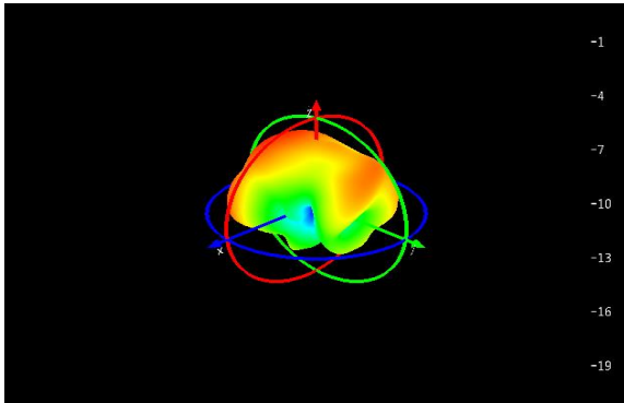
Ant0: 1900Mhz
