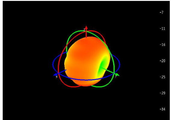
Ant0: 800Mhz
