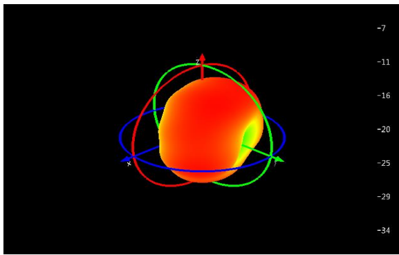
Ant0: 900Mhz
