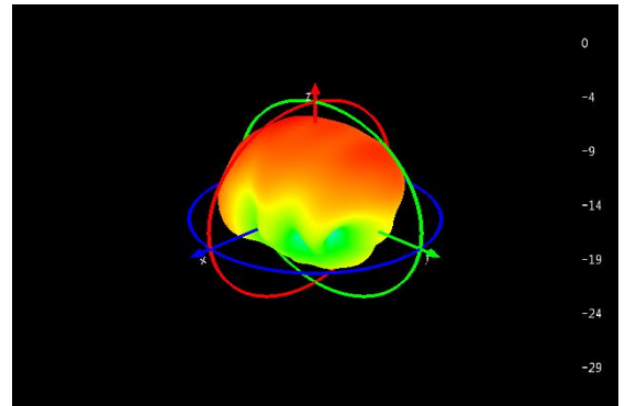
Ant0: 2600Mhz
