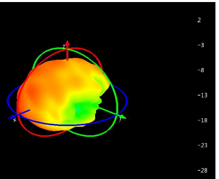
Ant2: 5500Mhz
