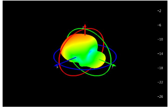
Ant0: 1700Mhz
