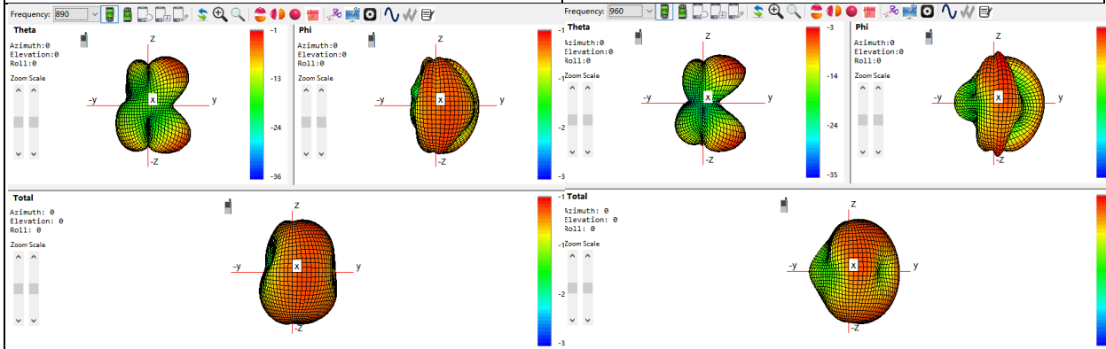
Main: 890Mhz
