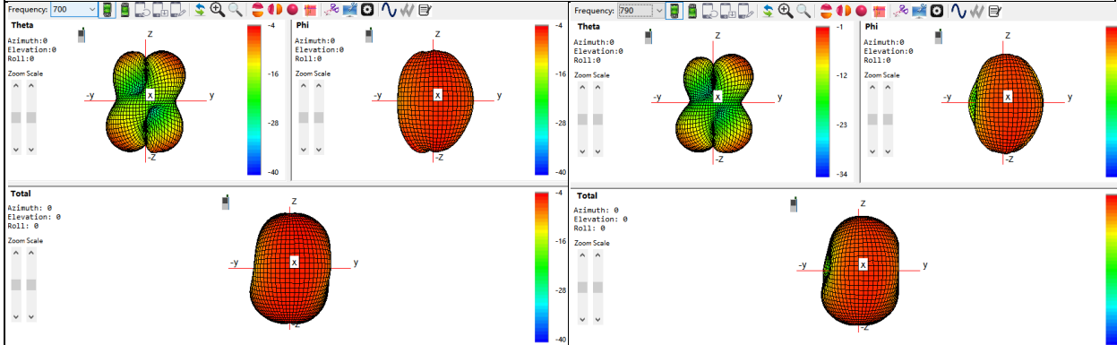
Main: 700Mhz
