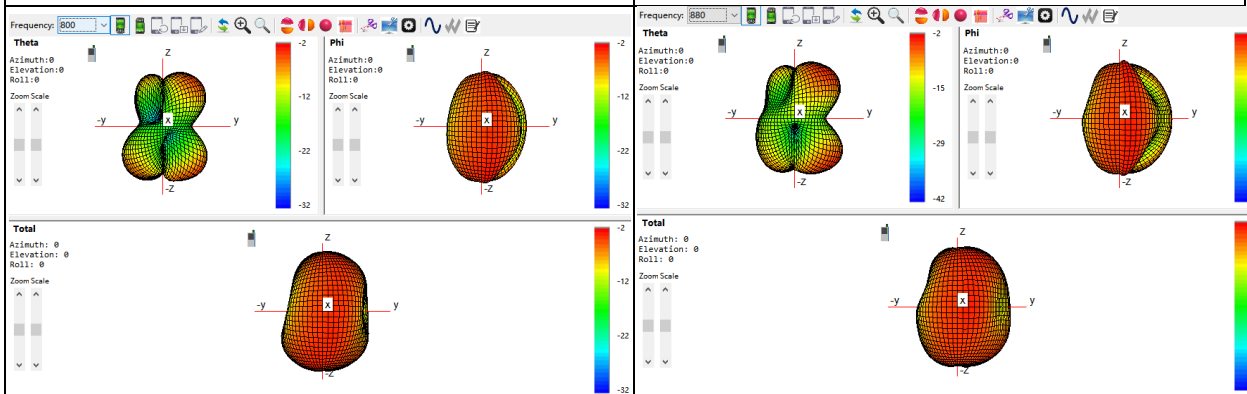
Main: 800Mhz
