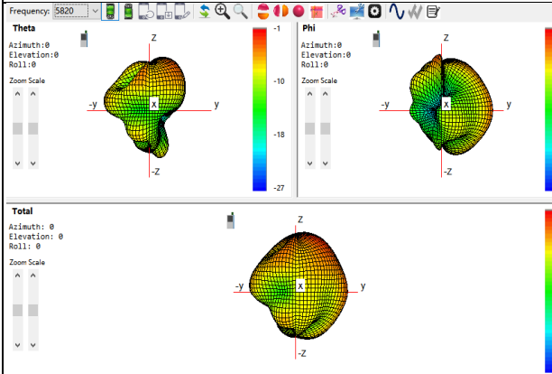
G/W/B: 5820Mhz
