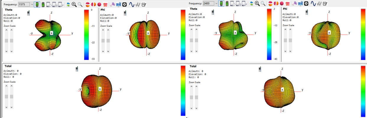
G/W/B: 1575Mhz
