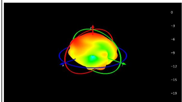
Ant0: 2100Mhz
