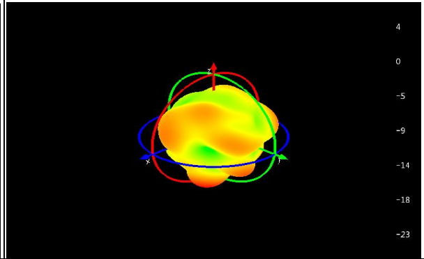
Ant0: 1700Mhz
