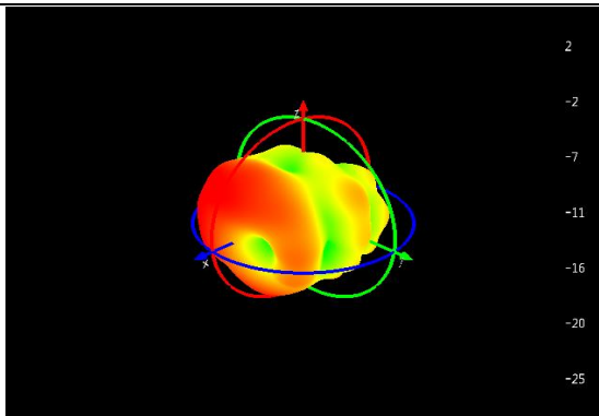
Ant7: 2450Mhz
