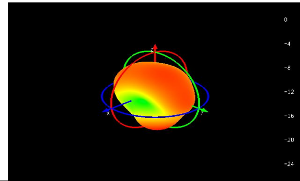
Ant0: 900Mhz
