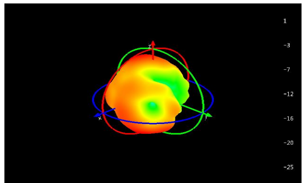
Ant0: 2400Mhz
