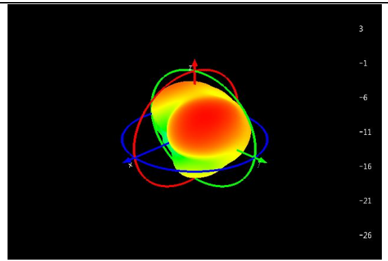
Ant7: 5500Mhz
