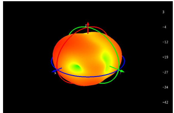
Ant7: 1575Mhz
