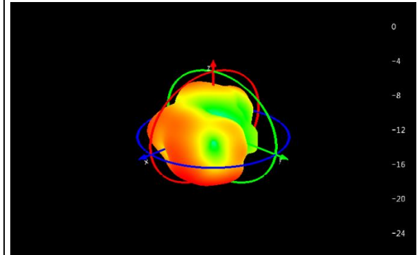
Ant0: 2600Mhz
