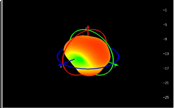
Ant0: 800Mhz
