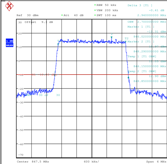
Band26(824-849)-3MHz-QPSK-26915-15RB#0-P ASS
