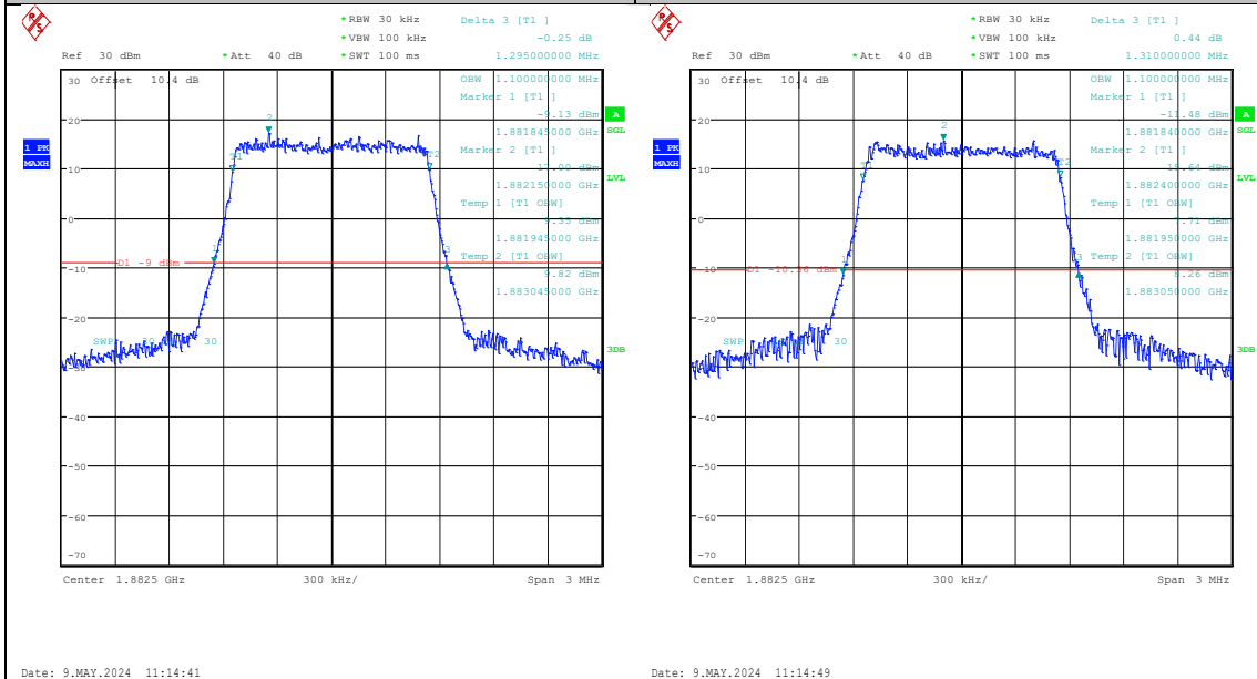
Band25-1.4MHz-QPSK-26365-6RB#0-PASS Band25-1.4MHz-16QAM-26365-6RB#0-PASS
