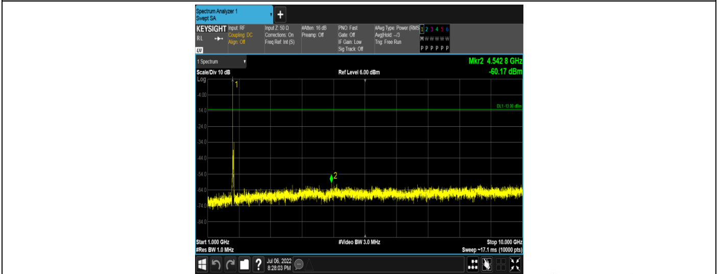
Band66-20MHz-QPSK-132072-1RB#0-Range3:1000~10000MHz
