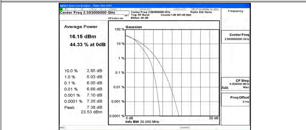
Band41-20MHz-QPSK-41490-1RB#0
