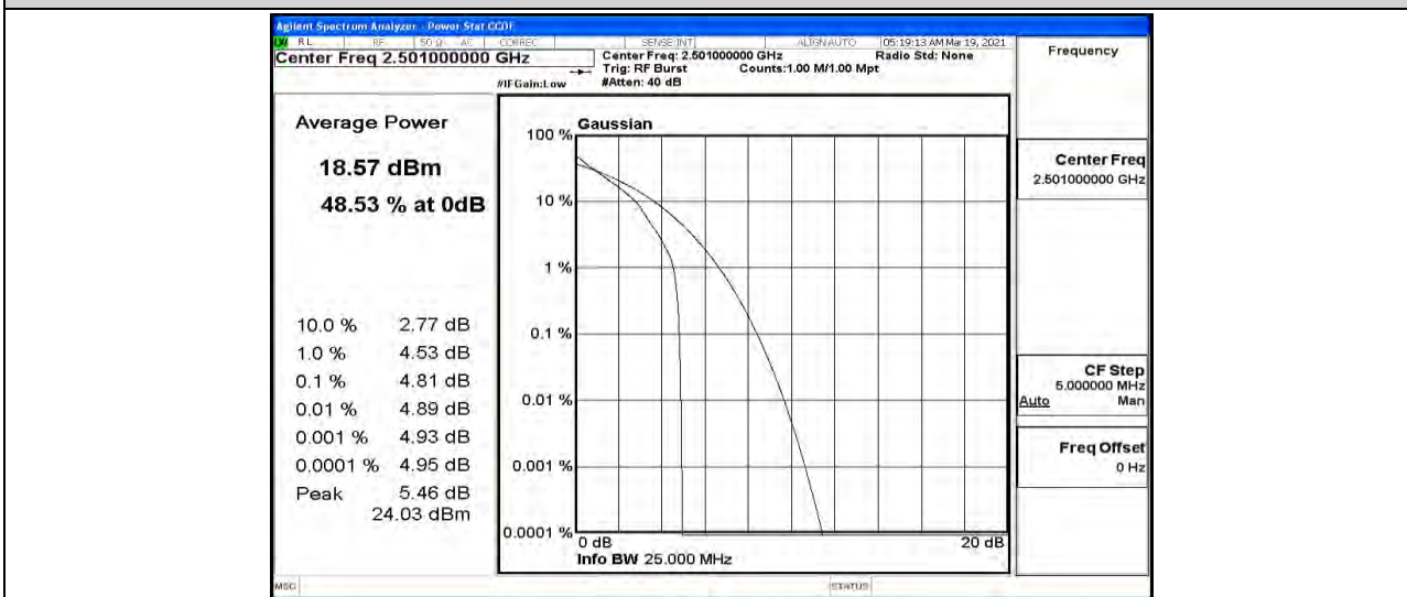
Band41-10MHz-QPSK-39700-50RB#0
