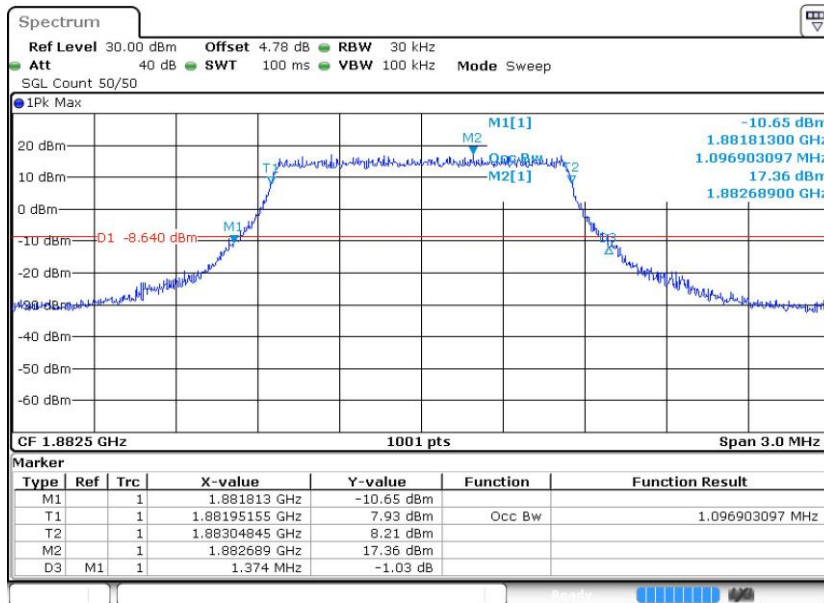
Band25-1.4MHz-QPSK-26365-6RB#0
