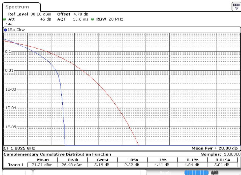
Band25-20MHz-QPSK-26365-100RB#0
