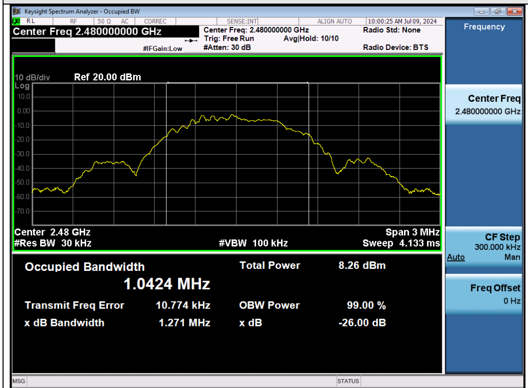
Test_Graph_2.4G_ANT1_2480_OBW
