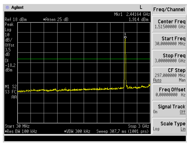
30MHz-3GHz
