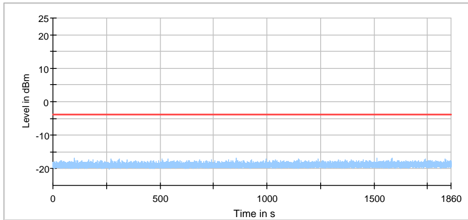
IEEE 802.11n HT40 5270MHz
