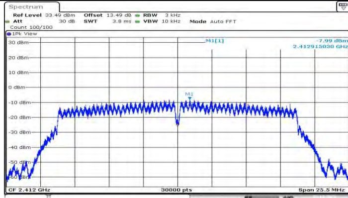
11N20MIMO Ant1 2412
