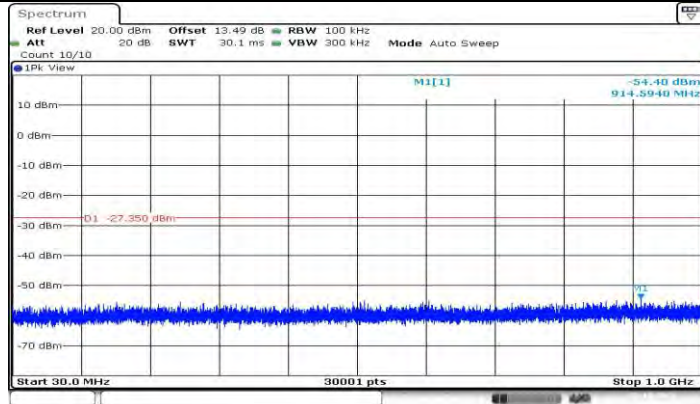
11N40MIMO_Ant2_2422_0~Reference
