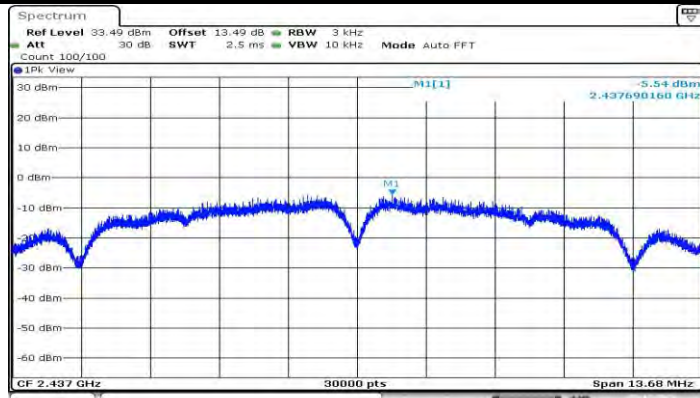
11B_Ant2_2437
