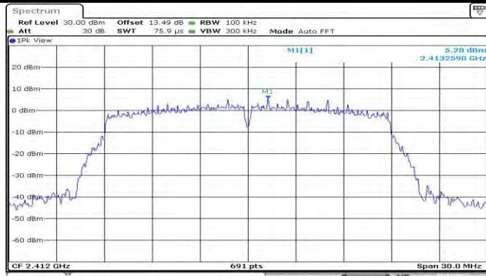
11N20MIMO_Ant2_2412_0~Reference
