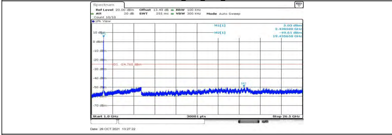
11N20MIMO_Ant2_2437_1000~26500
