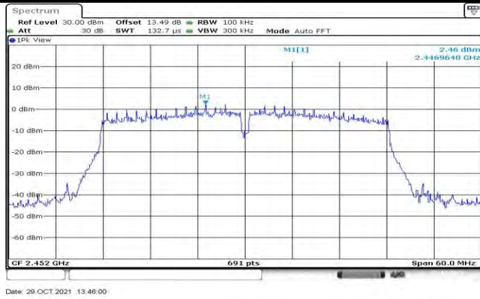
11N40MIMO_Ant2_2452_0~Reference
