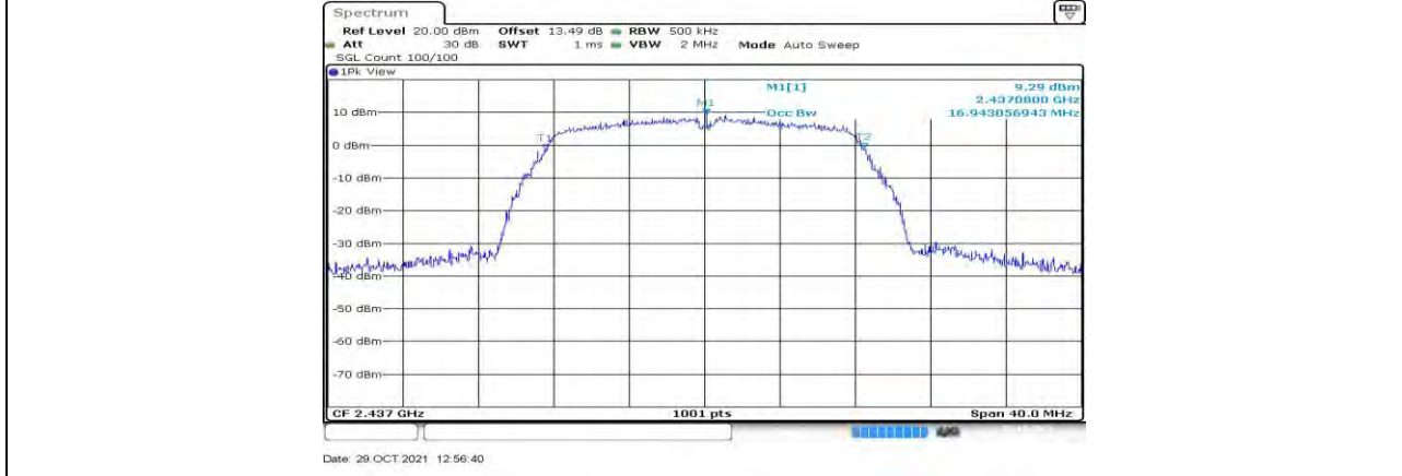
11G Ant1 2437
