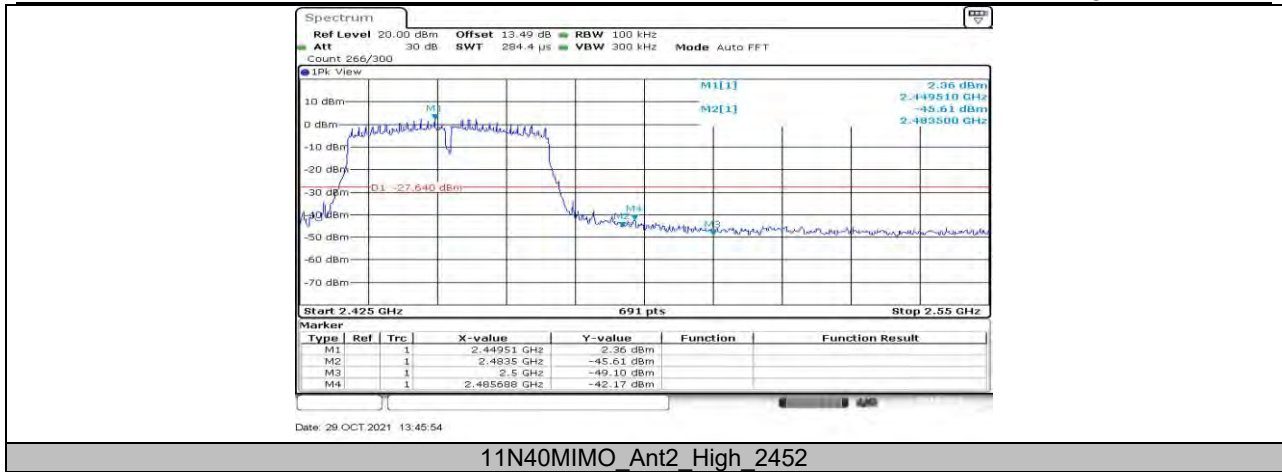
11N40MIMO_Ant2_High_2452
