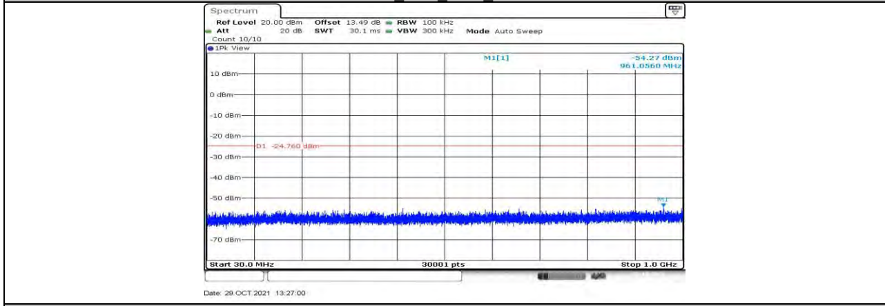
11N20MIMO_Ant2_2437_30~1000
