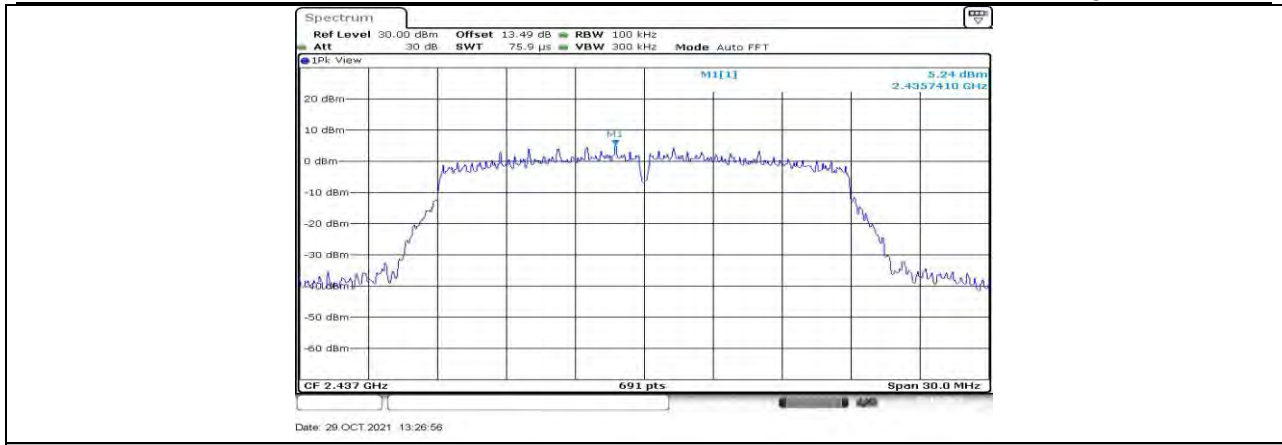
11N20MIMO_Ant2_2437_0~Reference
