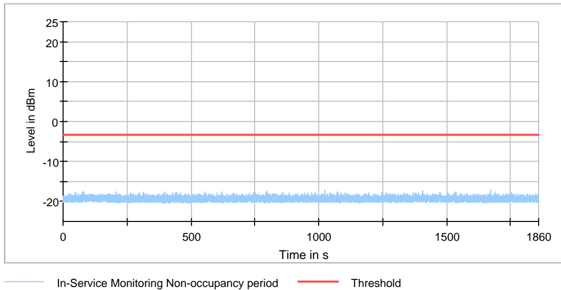
802.11a 5260MHz
