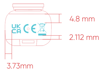
底部视图
