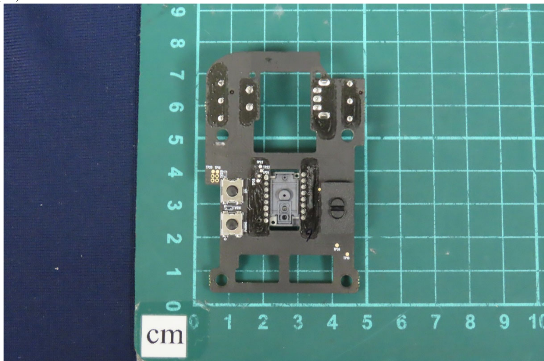
(13) EUT Photo
