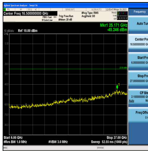
Band7-20MHz-QPSK-21100-100RB#0-Range3:6000~27000MHz
