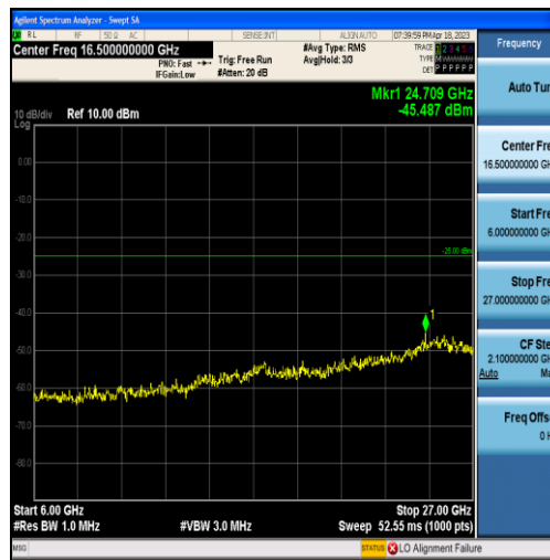
Band7-10MHz-16QAM-20800-50RB#0-Range3:6000~27000MHz
