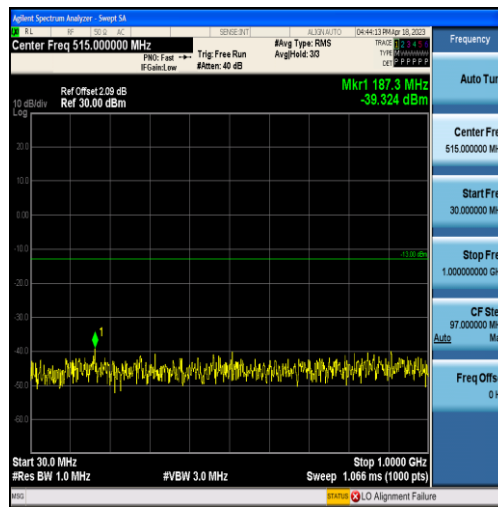
Band4-1.4MHz-QPSK-20393-6RB#0-Range1:30~1000MHz
