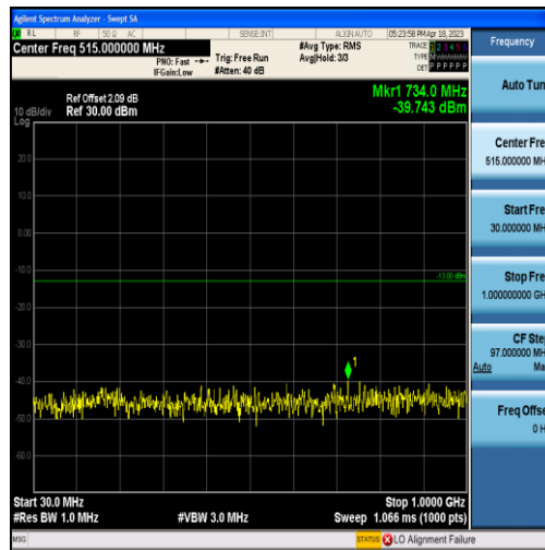
Band4-10MHz-QPSK-20000-50RB#0-Range1:30~1000MHz
