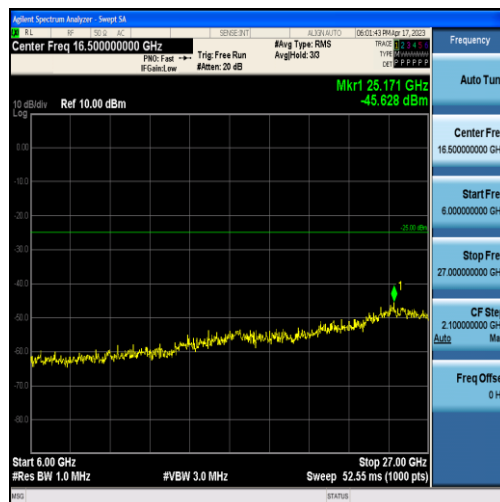
Band7-20MHz-QPSK-21350-60RB#0-Range3:6000~27000MHz
