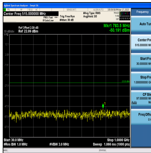
Band7-20MHz-QPSK-20850-60RB#0-Range1:30~1000MHz
