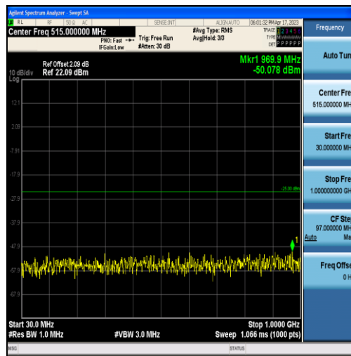
Band7-20MHz-QPSK-21350-60RB#0-Range1:30~1000MHz
