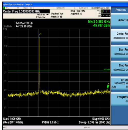
Band7-20MHz-QPSK-21100-60RB#0-Range2:1000~6000MHz
