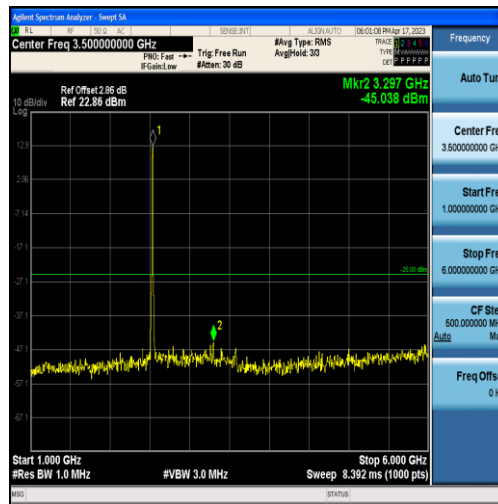
Band7-20MHz-16QAM-21100-60RB#0-Range2:1000~6000MHz
