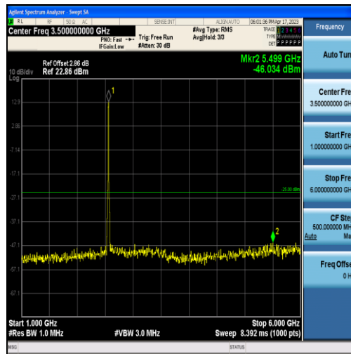
Band7-20MHz-QPSK-21350-60RB#0-Range2:1000~6000MHz
