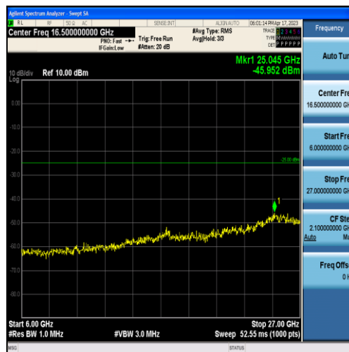
Band7-20MHz-16QAM-21100-60RB#0-Range3:6000~27000MHz
