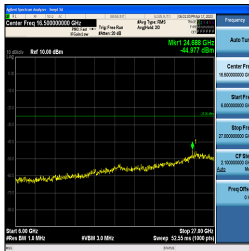
Band7-20MHz-QPSK-21100-60RB#0-Range3:6000~27000MHz
