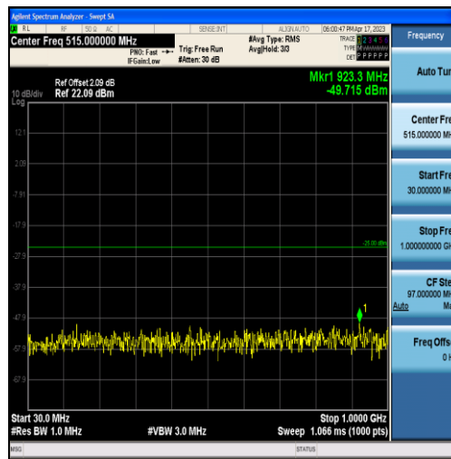
Band7-20MHz-QPSK-21100-60RB#0-Range1:30~1000MHz
