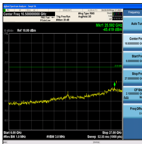
Band7-20MHz-QPSK-20850-60RB#0-Range3:6000~27000MHz
