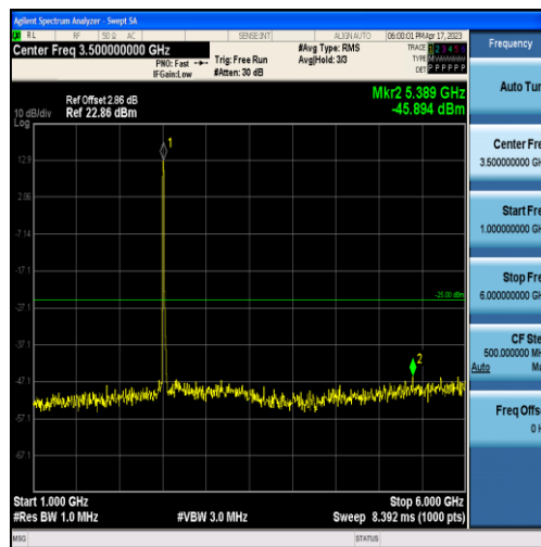
Band7-20MHz-QPSK-20850-60RB#0-Range2:1000~6000MHz
