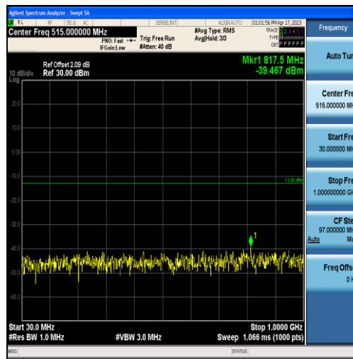
Band4-1.4MHz-QPSK-19957-6RB#0-Range1:30~1000MHz
