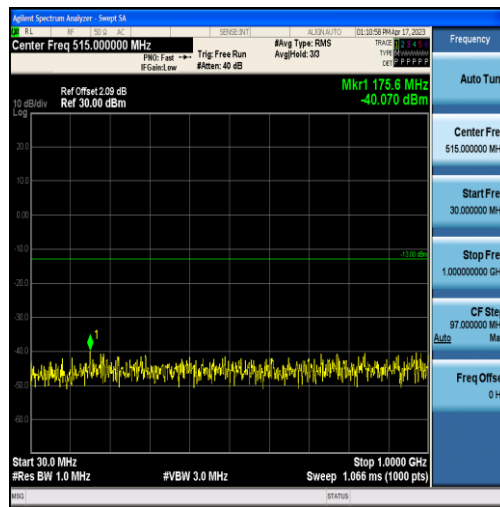
Band4-3MHz-QPSK-19965-15RB#0-Range1:30~1000MHz
