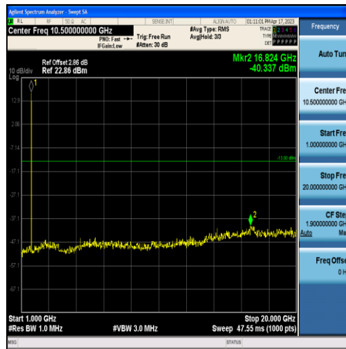
Band4-3MHz-QPSK-19965-15RB#0-Range2:1000~20000MHz
