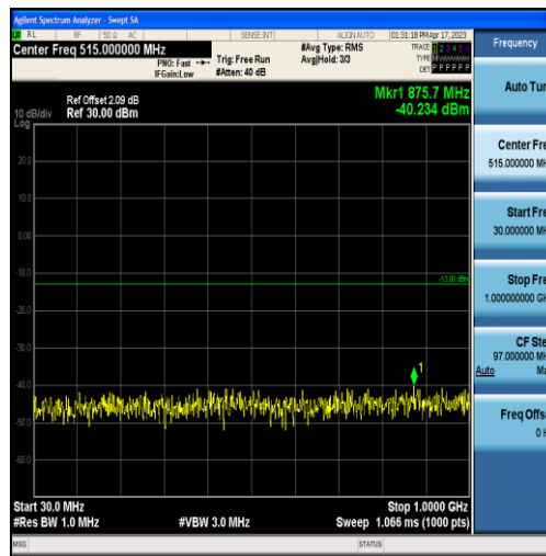
Band4-10MHz-QPSK-20000-50RB#0-Range1:30~1000MHz
