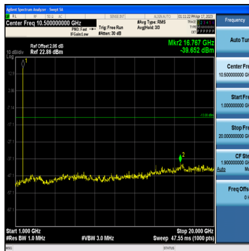
Band4-3MHz-QPSK-20175-15RB#0-Range2:1000~20000MHz
