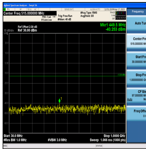
Band2-20MHz-QPSK-18700-100RB#0-Range1:30~1000MHz
