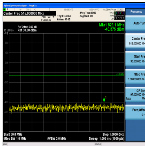
Band4-1.4MHz-QPSK-20393-6RB#0-Range1:30~1000MHz
